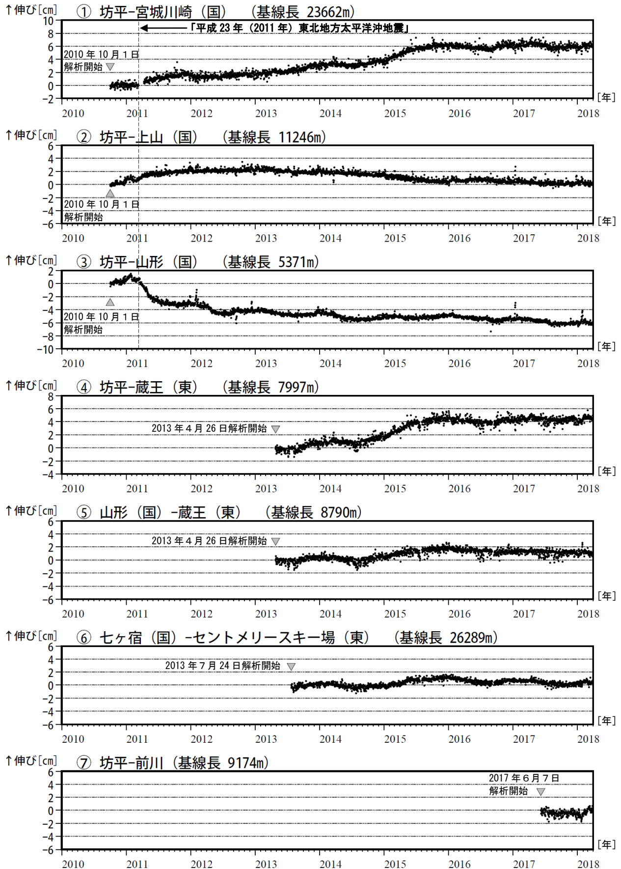
図 15 蔵王山 GNSS 基線長変化図 (2010 年 10 月～2018 年 3 月)
