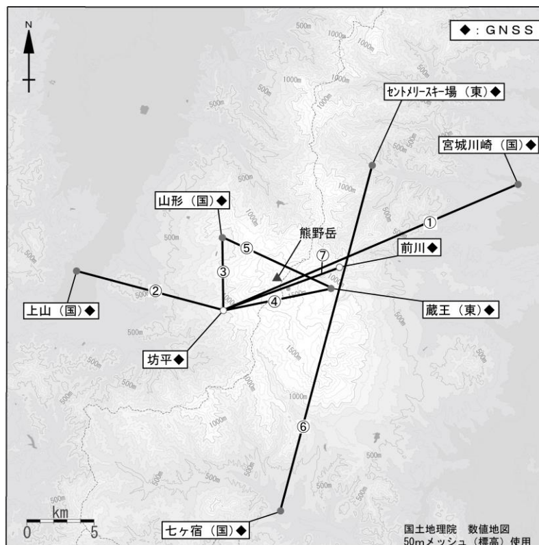
図 17 蔵王山 GNSS 観測点配置図
