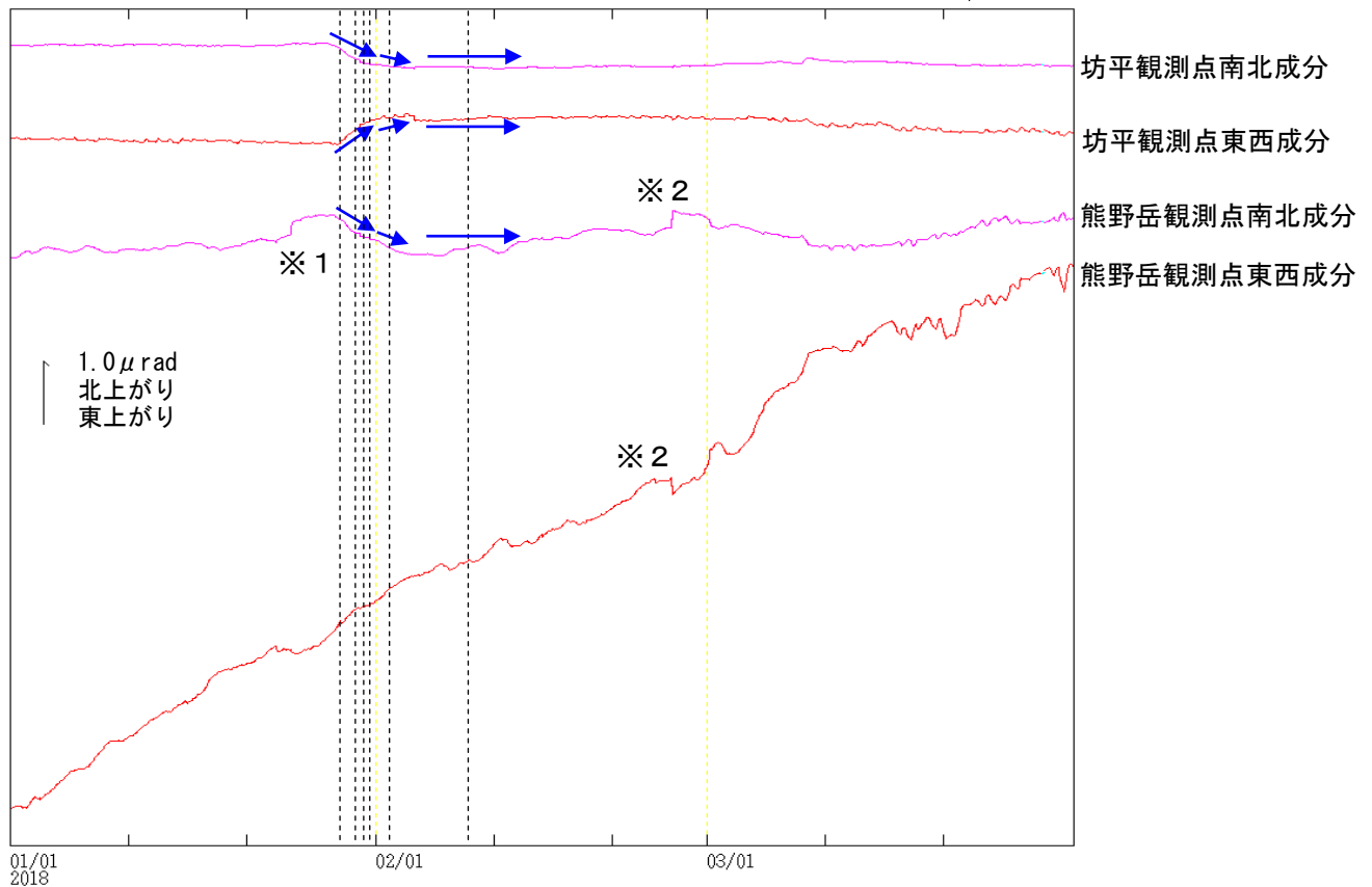
図 14 蔵王山 坊平観測点及び熊野岳観測点での傾斜変動 (2018 年 1 月 1 日 00 時 00 分～3 月 31 日 24 時 00 分)
