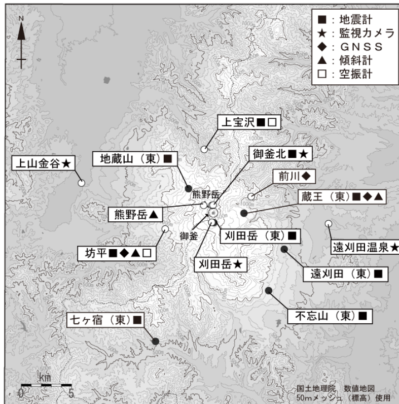
図 16 蔵王山 観測点配置図
