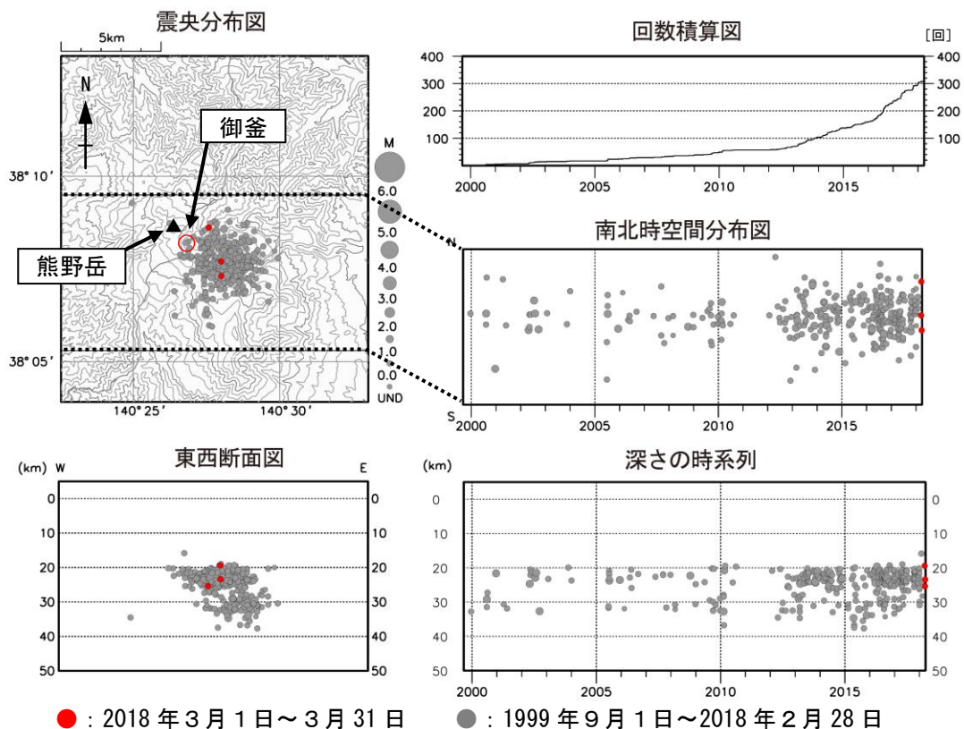
図 13 蔵王山 広域地震観測網による深部低周波地震活動（1999 年 9 月～2018 年 3 月）
