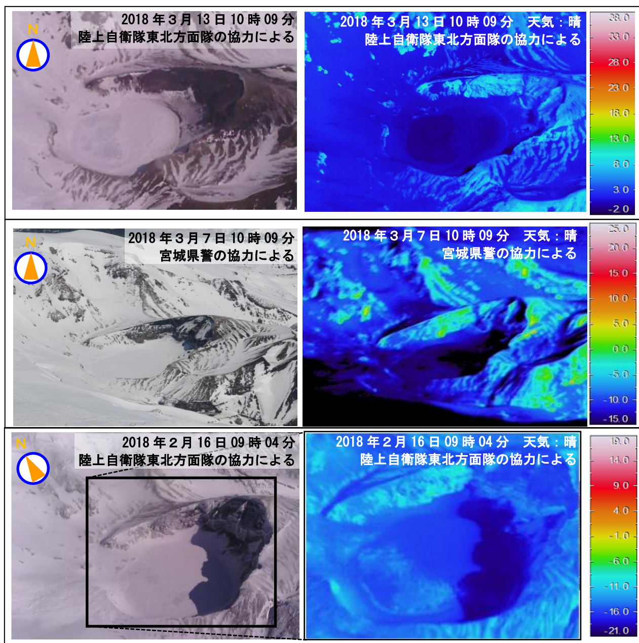
図 3 蔵王山 上空から撮影した御釜の状況と地表面温度分布
