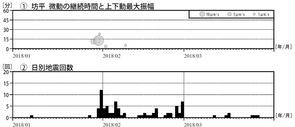
図11 蔵王山 微動の発生状況及び日別地震回数（2018年1月～2018年3月）
