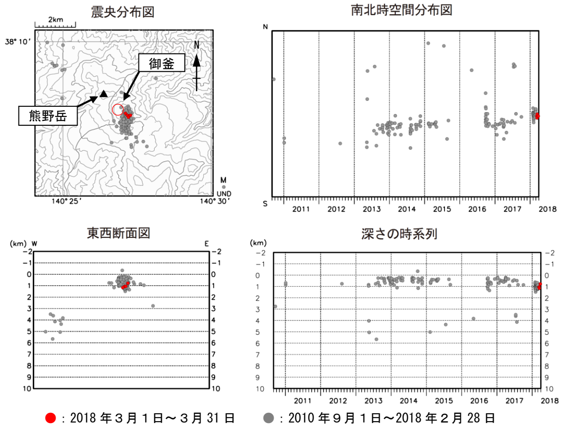
図 12 蔵王山 地震活動（2010 年 9 月～2018 年 3 月）
