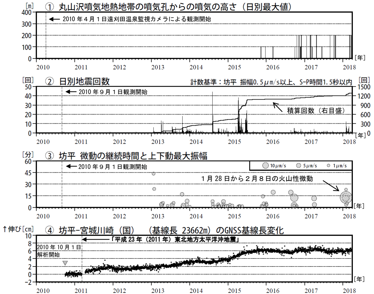
図10 蔵王山 火山活動経過図（2010年4月～2018年3月）
