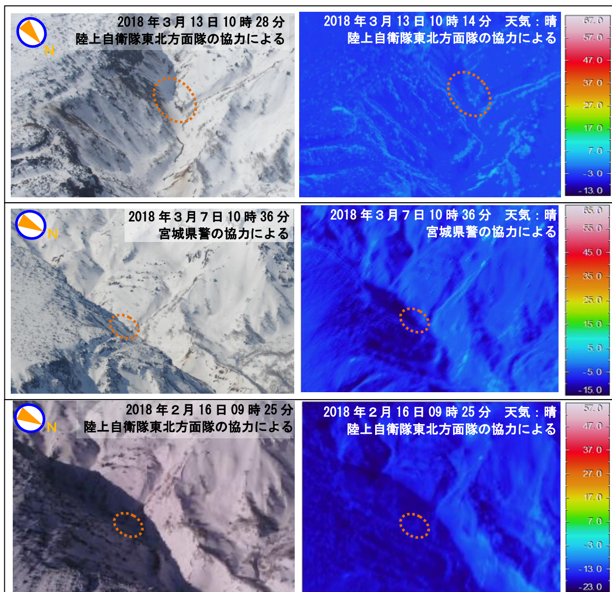
図 5 蔵王山 上空から撮影した振子沢付近の状況と地表面温度分布
