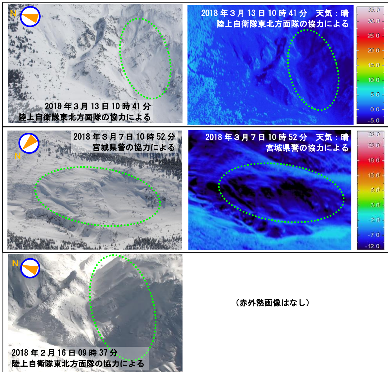
図 6 蔵王山 上空から撮影した傾城岩付近硫気変質地帯の状況と地表面温度分布
