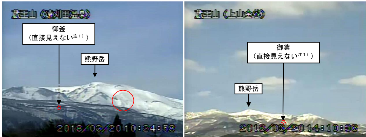
図 1 蔵王山 山頂部の状況
