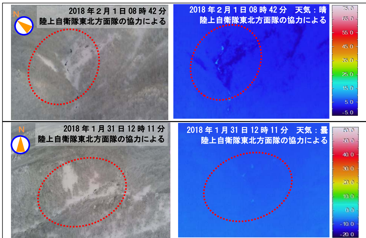
図6 蔵王山 上空から撮影した祓川上流域硫黄変質地帯の状況と地表面温度分布
