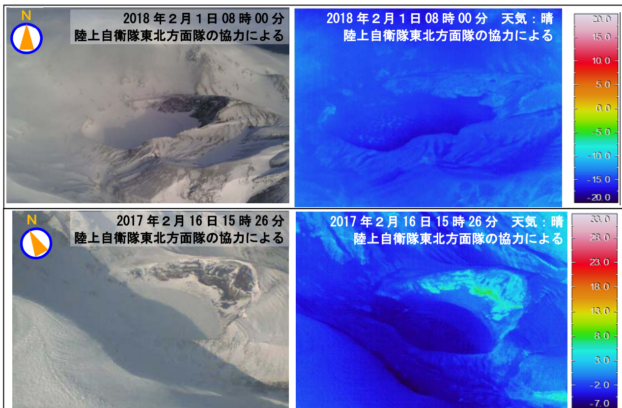
図2 蔵王山 上空から撮影した御釜の状況と地表面温度分布
