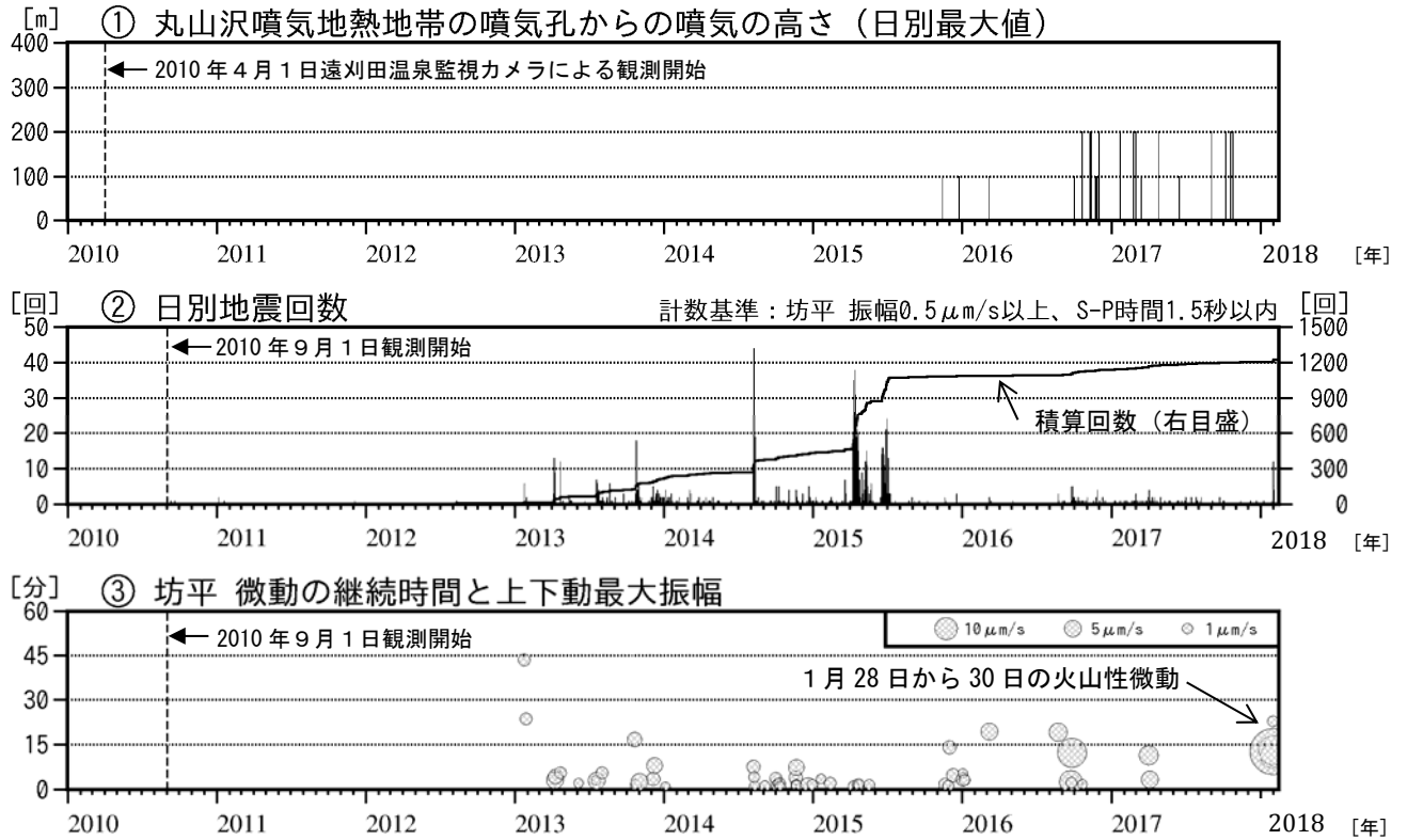
図9 蔵王山 火山活動経過図 (2010年4月～2018年2月1日)
