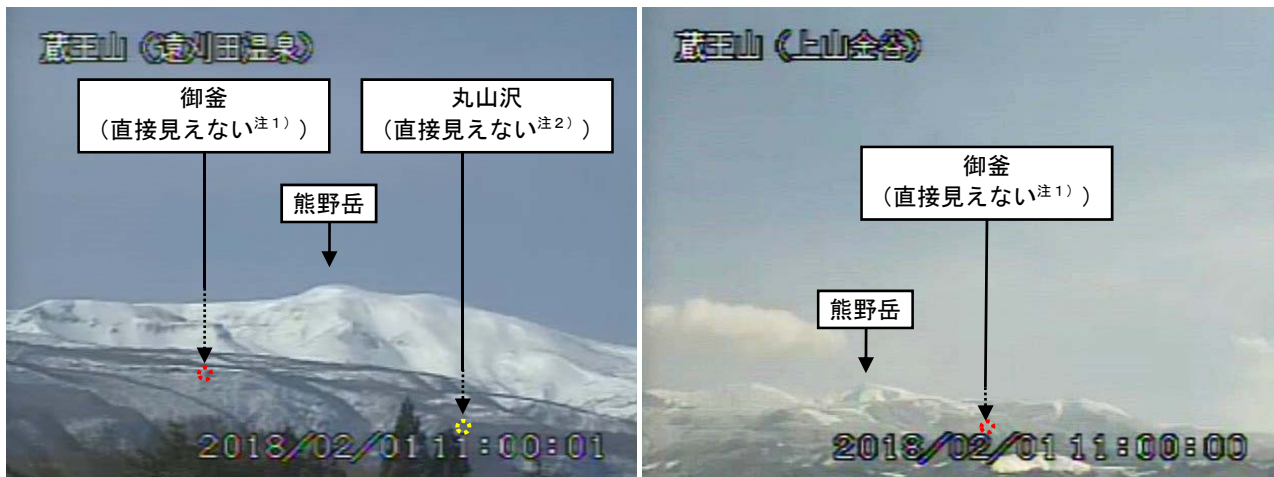
図7 蔵王山 山頂部の状況
