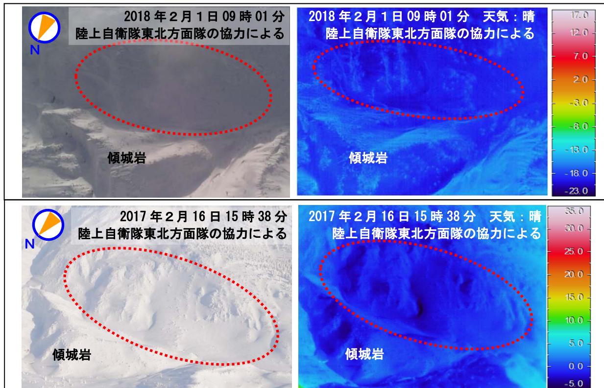
図5 蔵王山 上空から撮影した傾城岩付近硫黄変質地帯の状況と地表面温度分布
