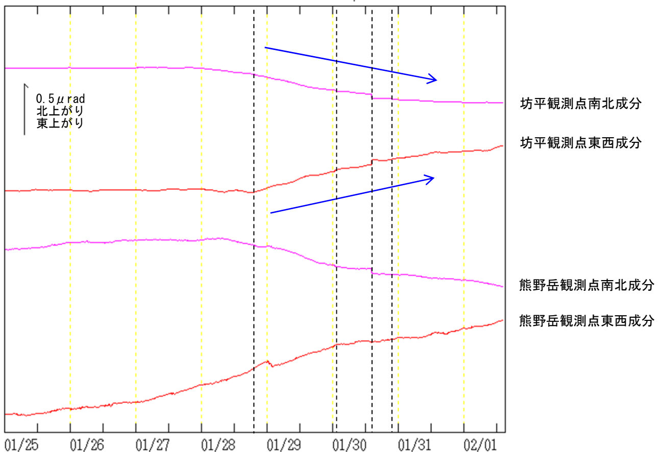
図8 蔵王山 坊平観測点及び熊野岳観測点での傾斜変動
