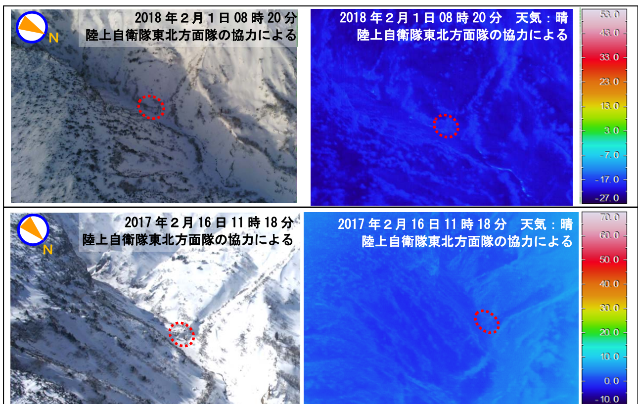
図4 蔵王山 上空から撮影した振り子沢付近の状況と地表面温度分布
