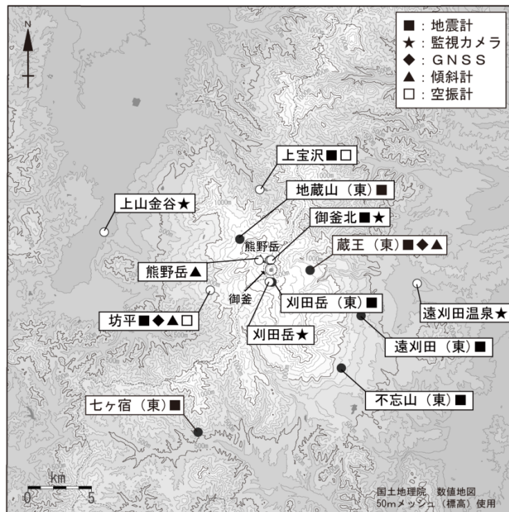
図 10 蔵王山 観測点配置図
