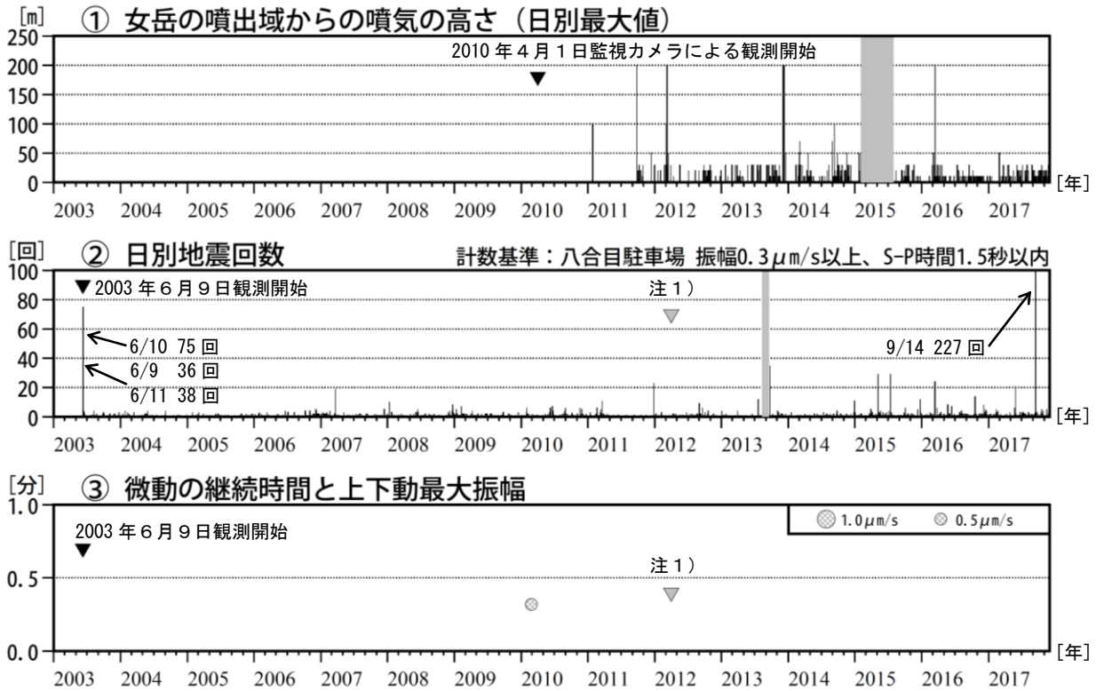
図5 秋田駒ヶ岳 火山活動経過図（2003年6月～2017年11月）
