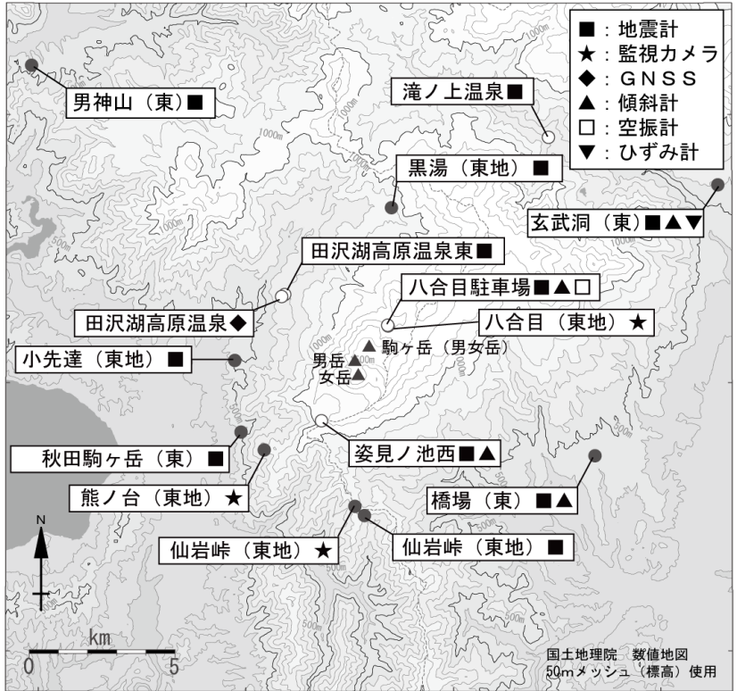
図7 秋田駒ヶ岳 観測点配置図
