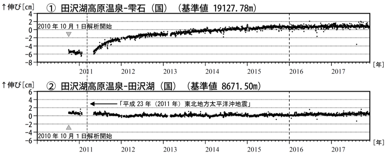
図6 秋田駒ヶ岳 GNSS 1) 基線長変化図（2010年10月～2017年11月）
