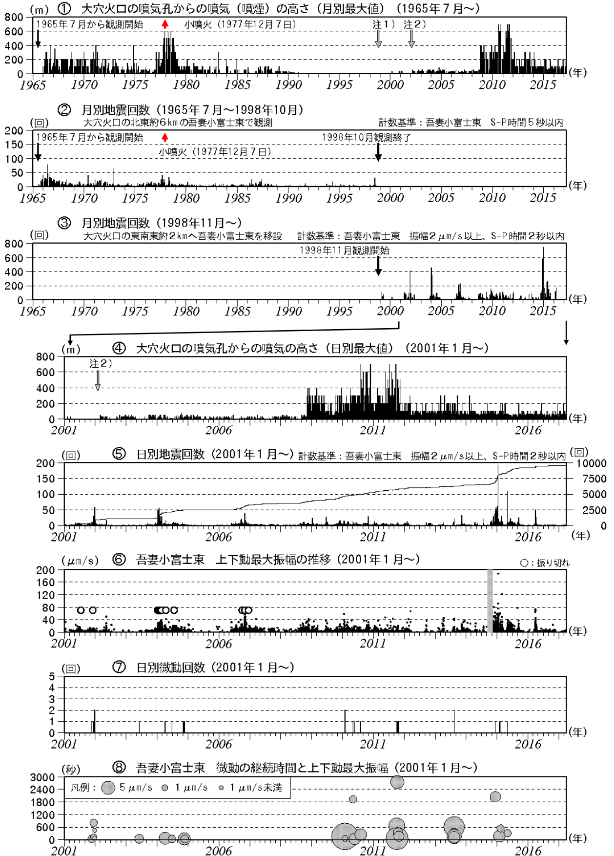
図2 吾妻山 火山活動経過図 (1965年7月～2017年3月)
