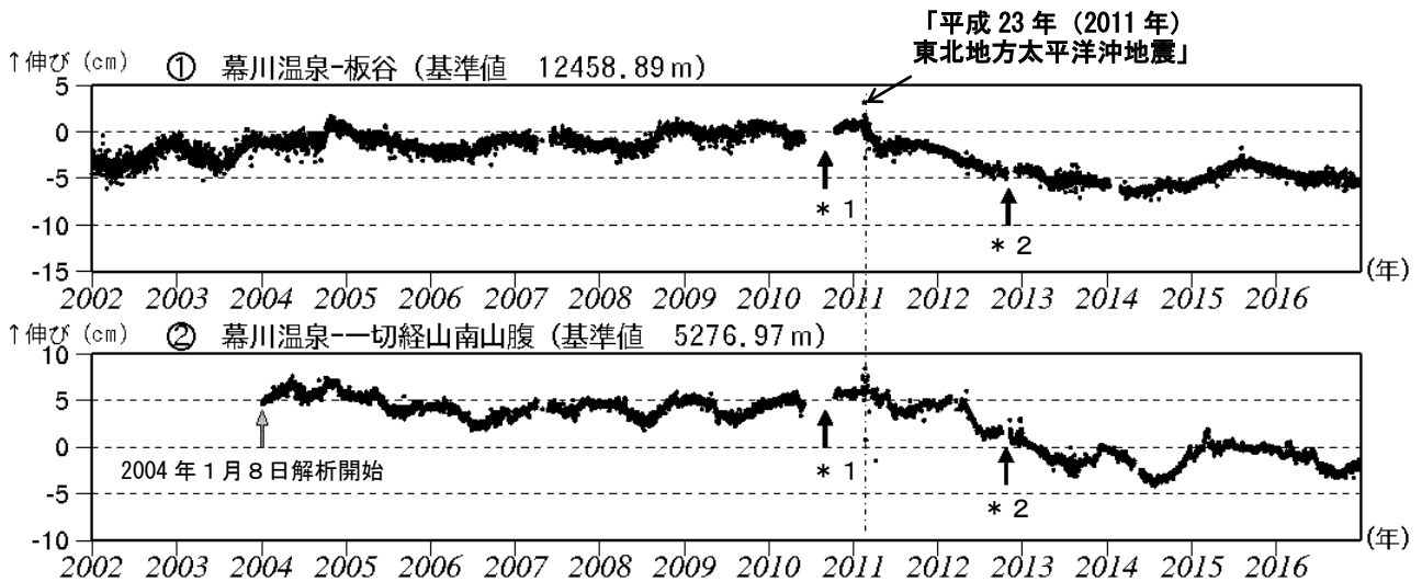
図4-1 吾妻山 GNSS 基線長変化図 (2002 年 1 月～2016 年 12 月)
