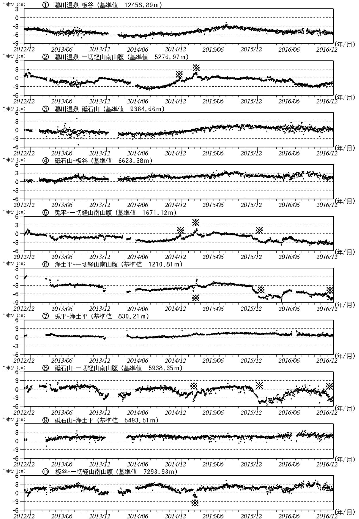
図 4-2 吾妻山 GNSS 基線長変化図 (2012 年 12 月～2016 年 12 月)
