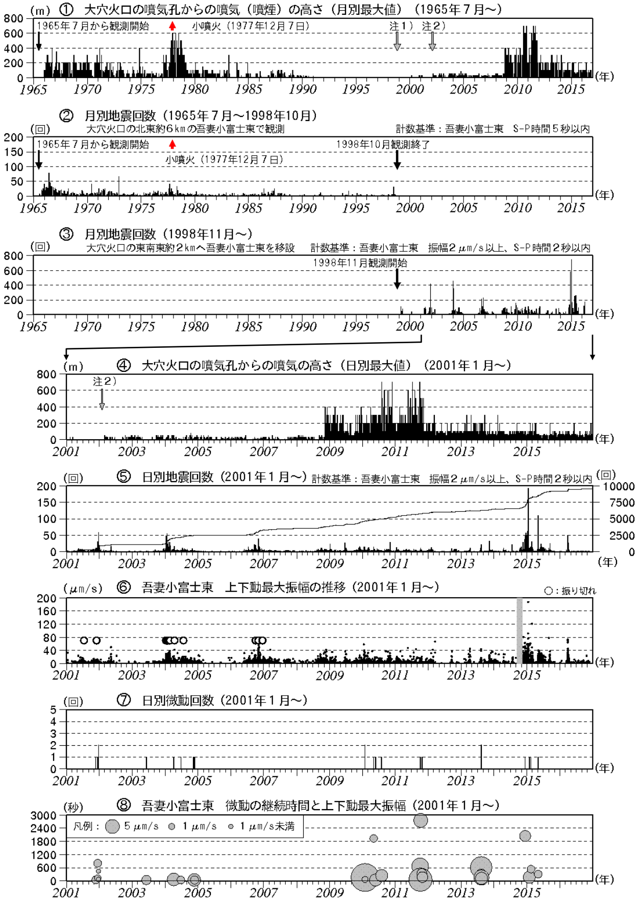
図2 吾妻山 火山活動経過図(1965年7月~2016年12月)
