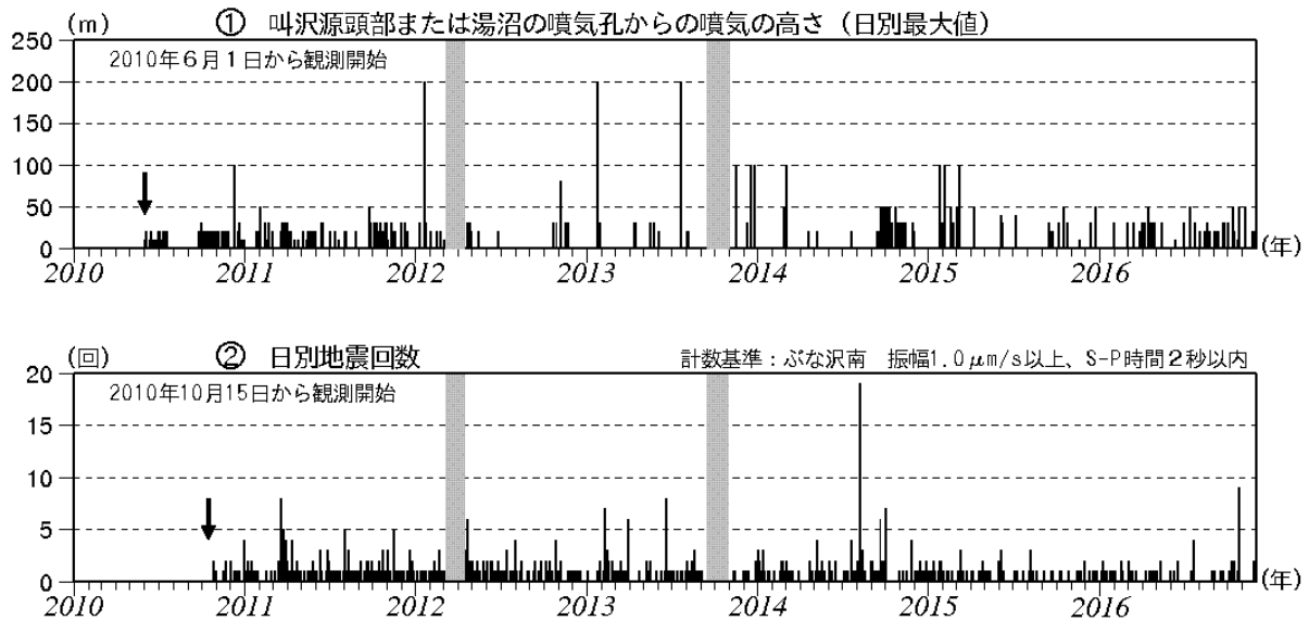
図3 秋田焼山 火山活動経過図（2010年6月～2016年11月）
