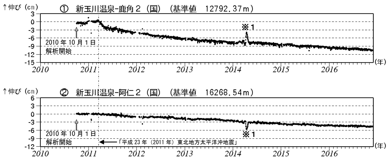
図4 秋田焼山 GNSS 1) 基線長変化図（2010年10月～2016年11月）
