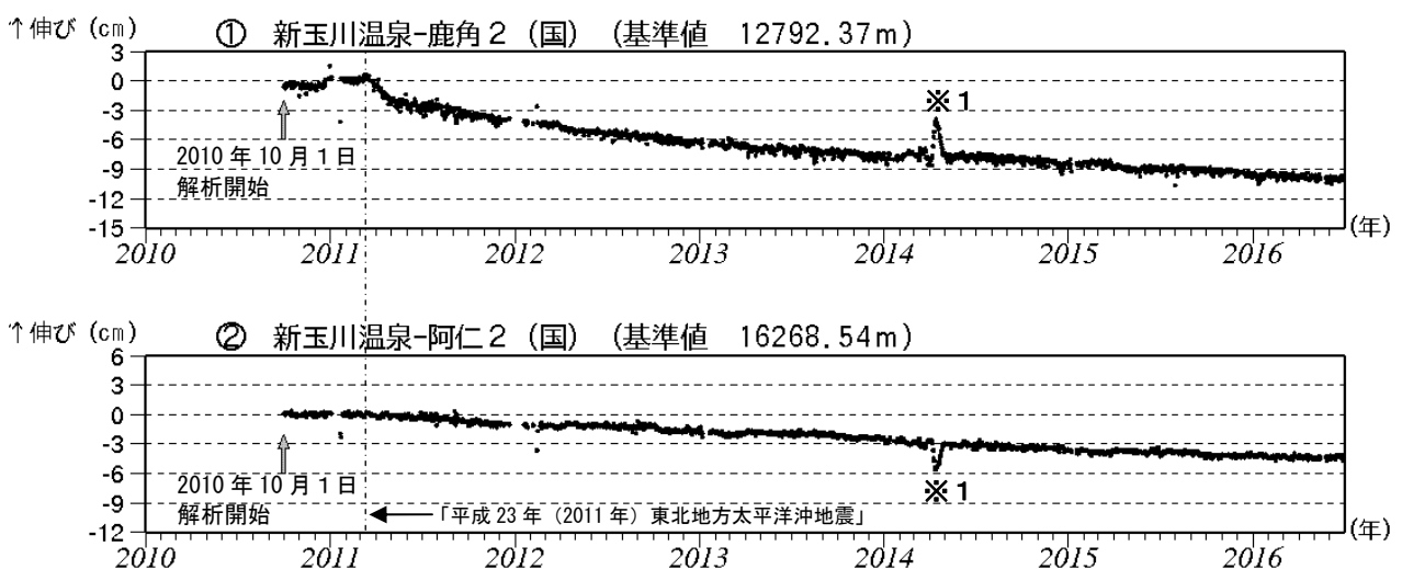
図4 秋田焼山 GNSS 1) 基線長変化図（2010年10月～2016年6月）
