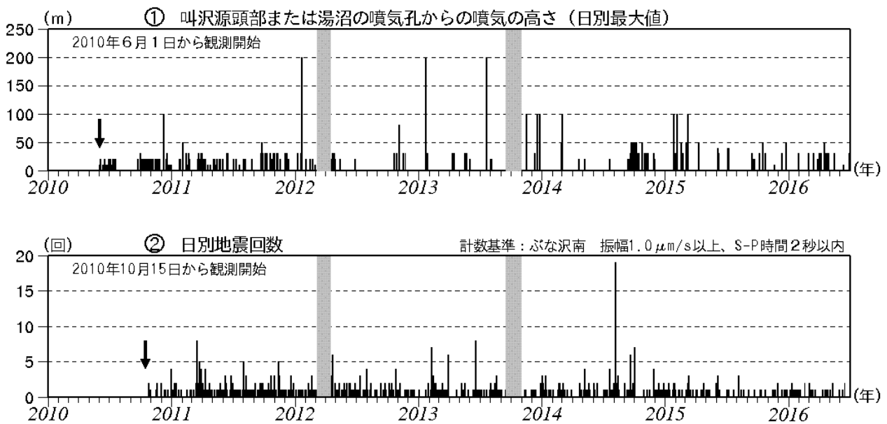
図3 秋田焼山 火山活動経過図（2010年6月～2016年6月）
