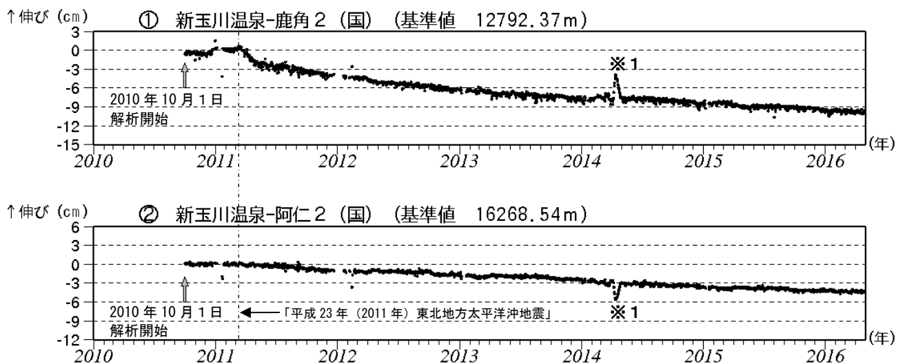
図3 秋田焼山 GNSS 1) 基線長変化図（2010年10月～2016年4月）
