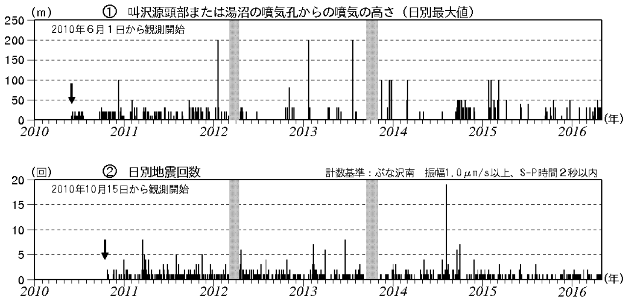
図2 秋田焼山 火山活動経過図（2010年6月～2016年4月）
