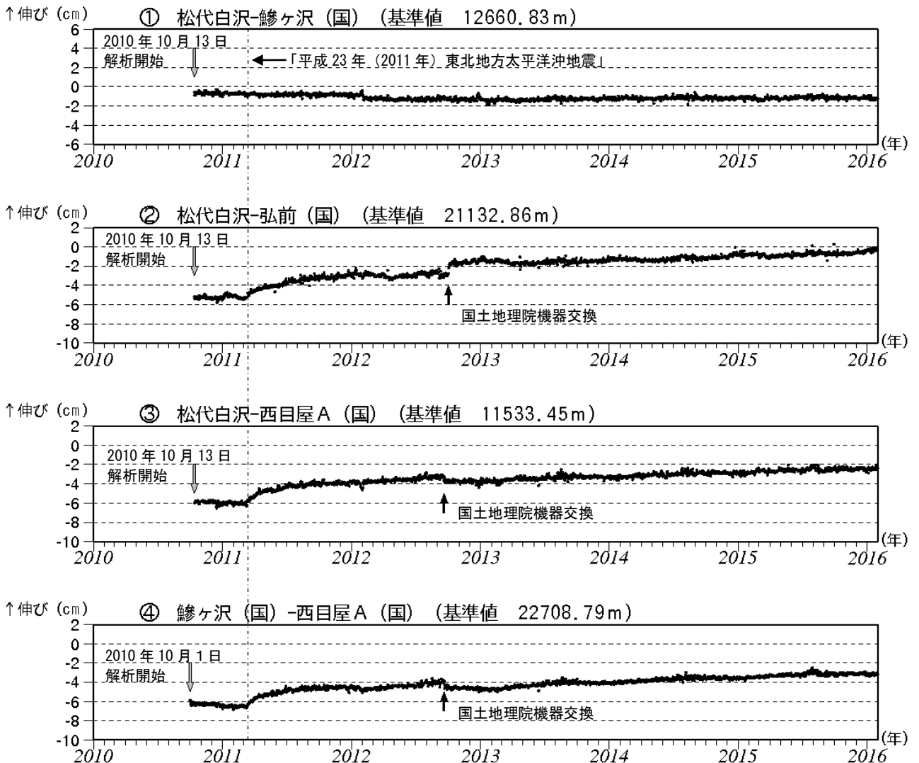
図3 岩木山 GNSS 1) 基線長変化図（2010年10月～2016年1月）
