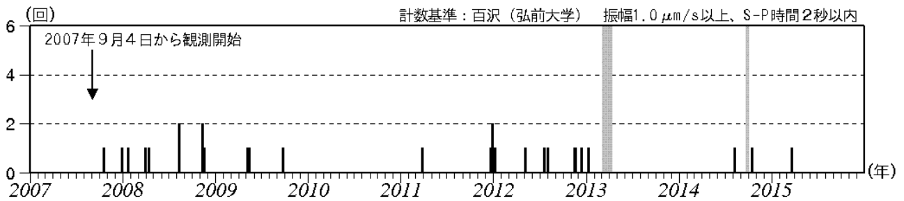
図2 岩木山 日別地震回数（2007年9月～2015年12月）
