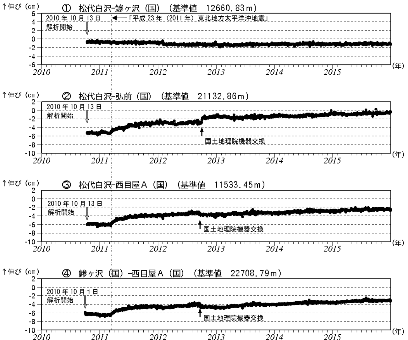
図3 岩木山 GNSS 1) 基線長変化図（2010年10月～2015年12月）
