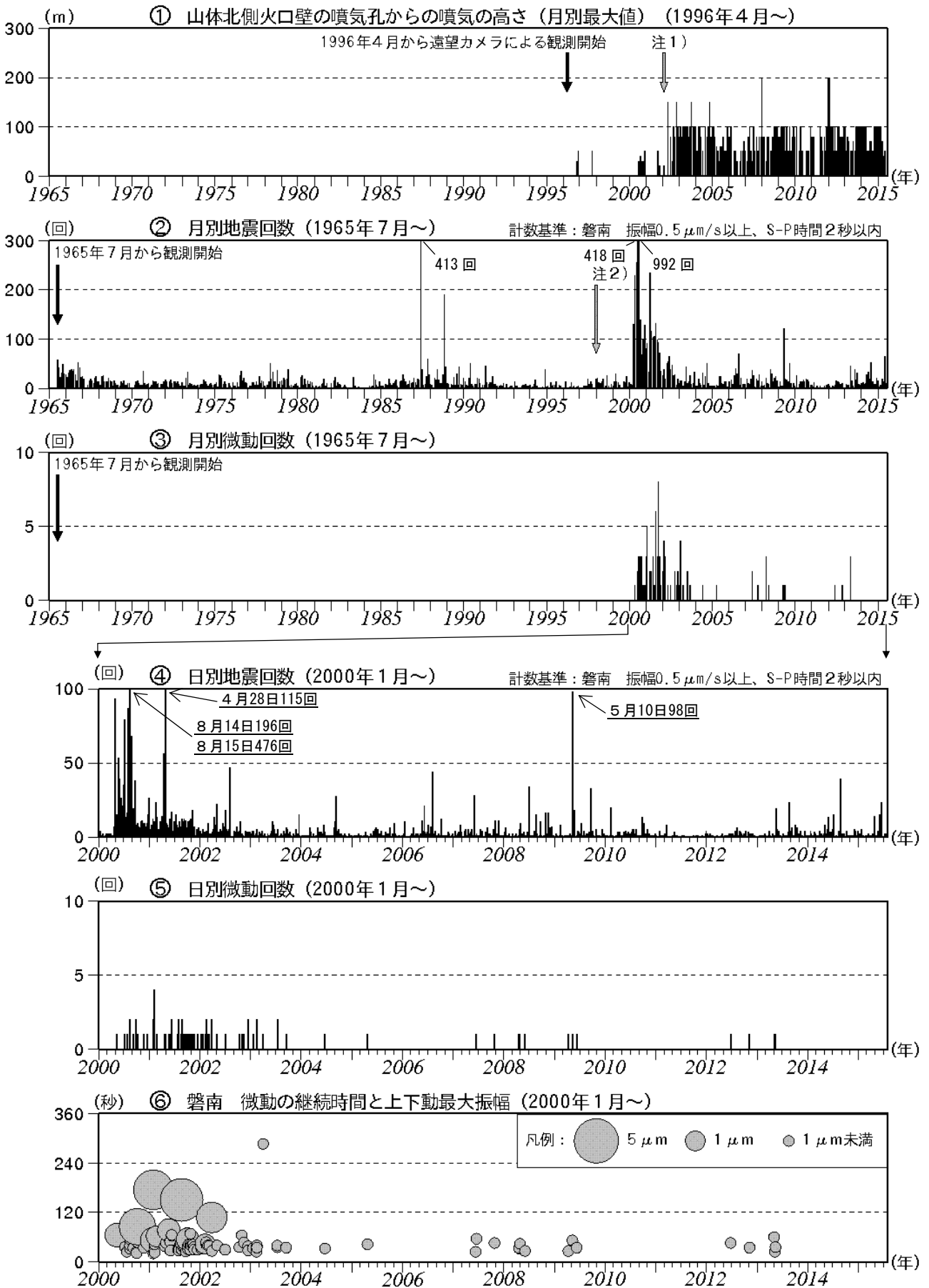
図2 磐梯山 火山活動経過図（1965年7月～2015年7月）
