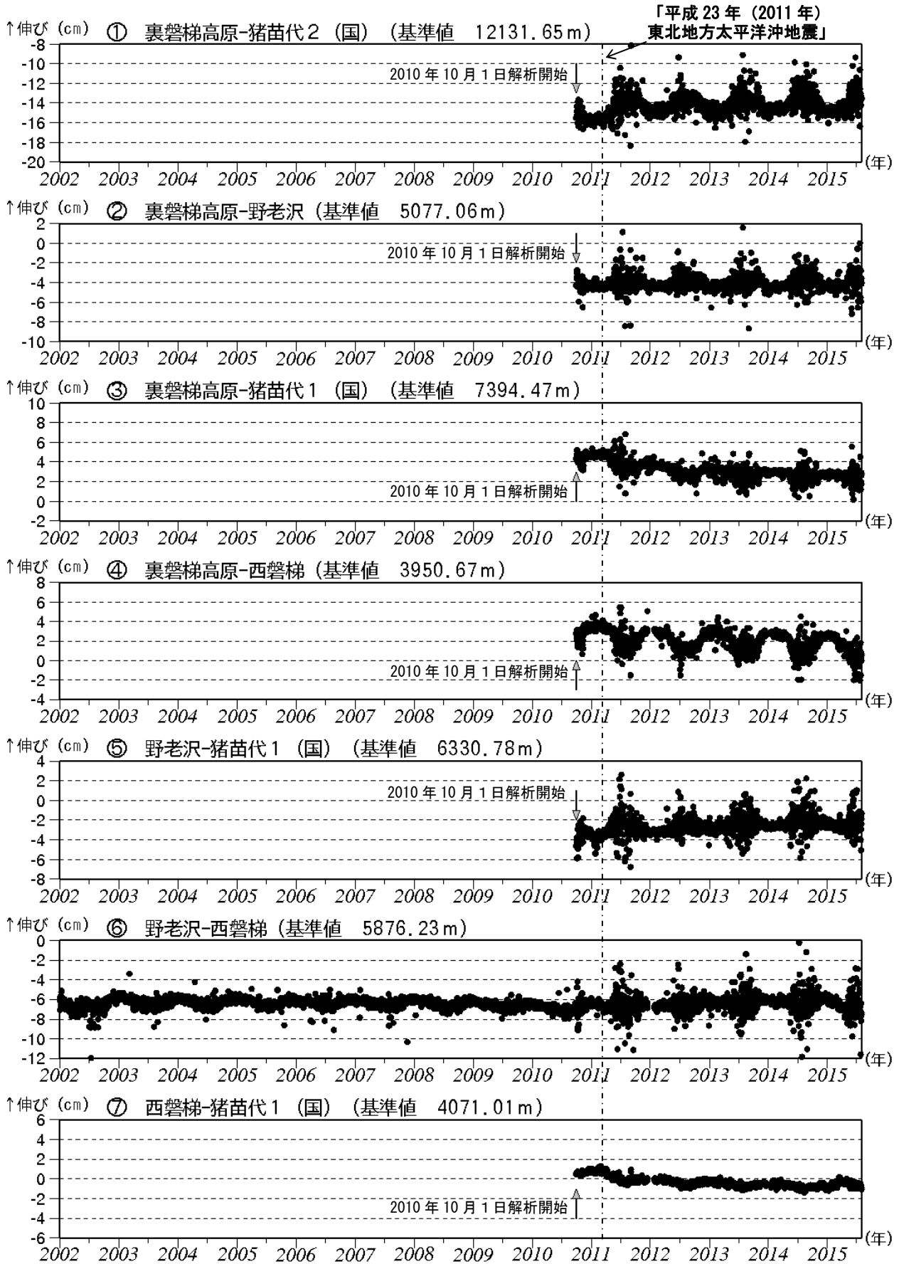
図3 磐梯山 GNSS 1) 基線長変化図 (2002 年 1 月~2015 年 7 月)
