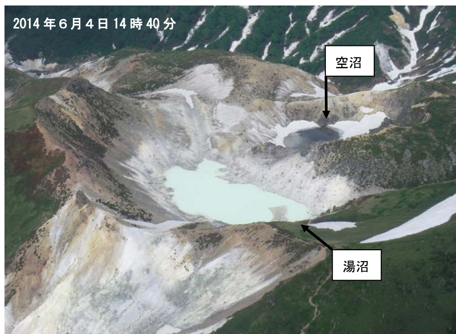
図 3 秋田焼山 湯沼及び空沼の可視画像
