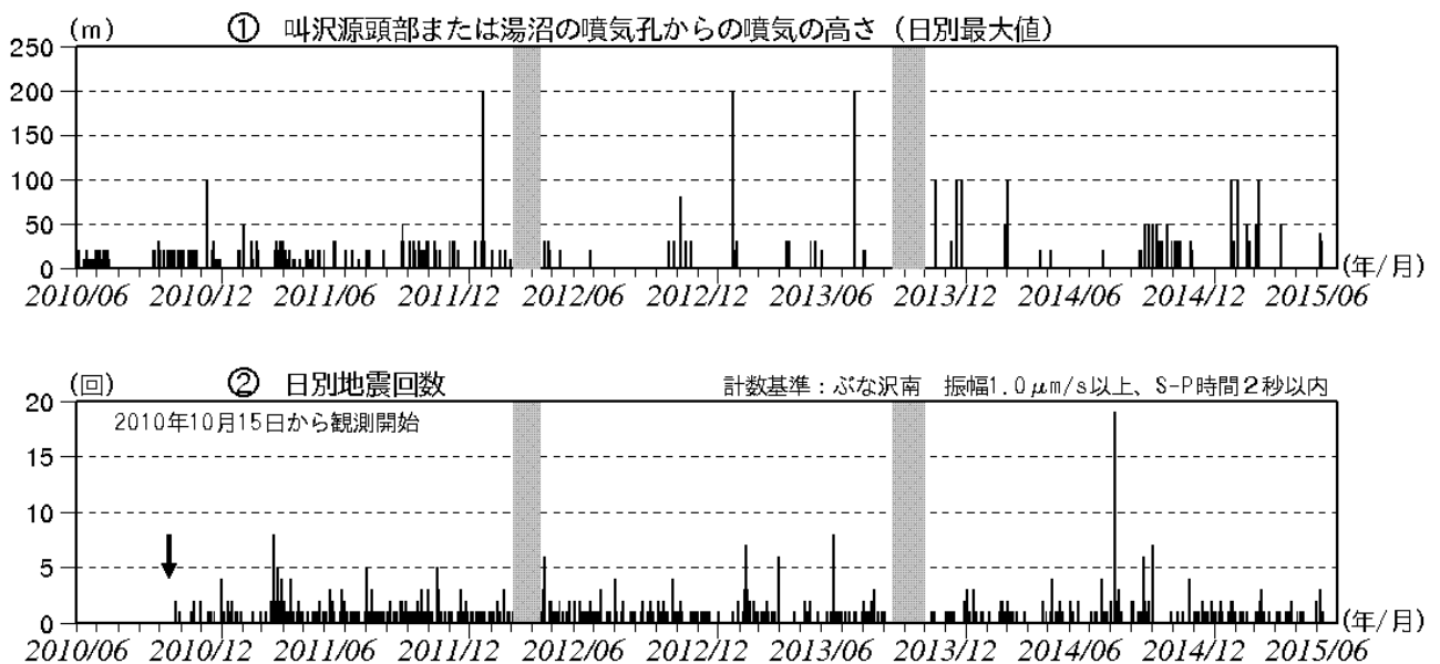
図4 秋田焼山 火山活動経過図（2010年6月～2015年6月）
