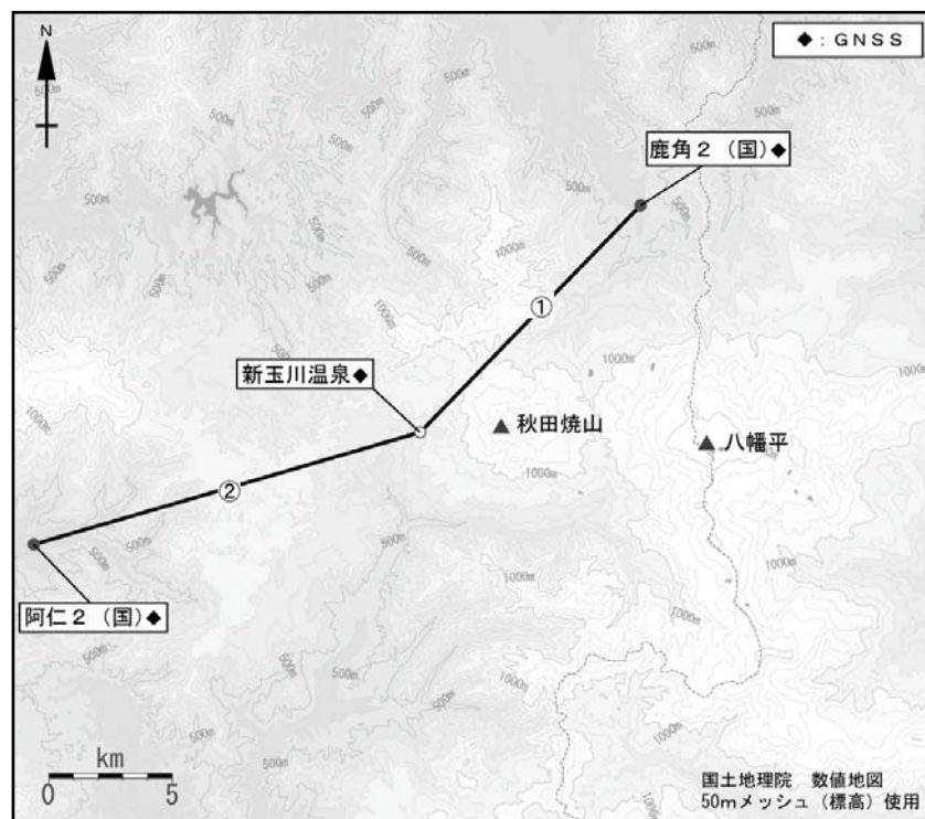
図7 秋田焼山 GNSS 観測点配置図
