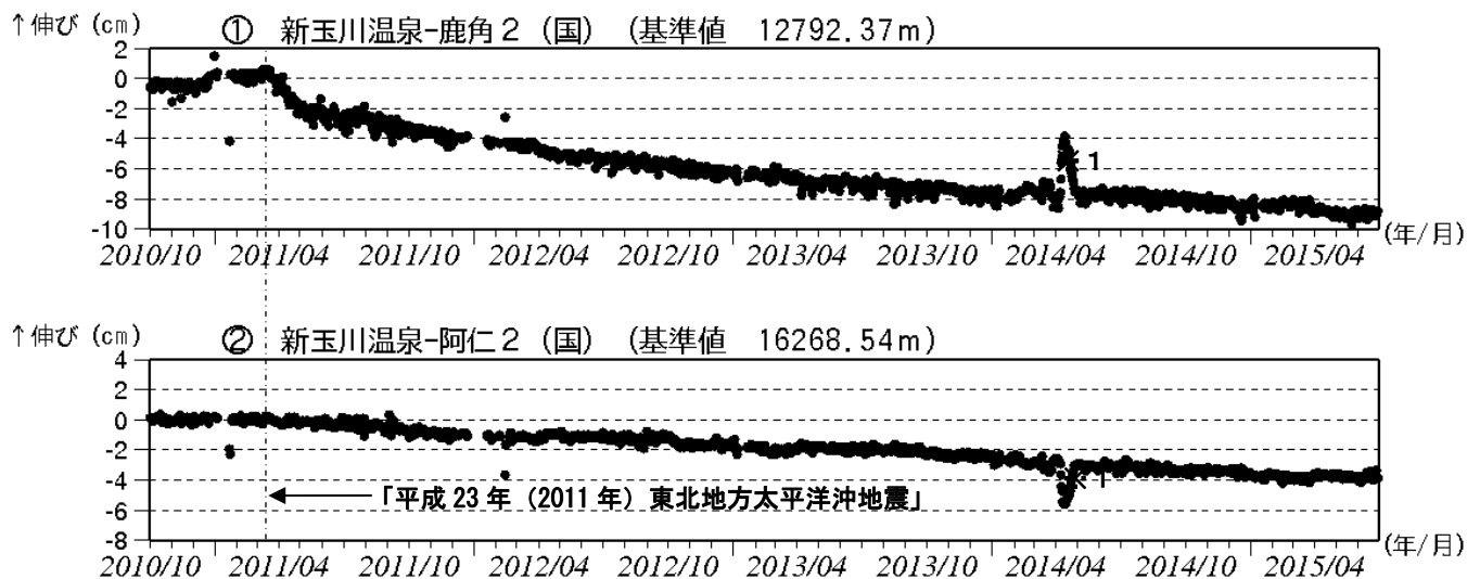
図5 秋田焼山 GNSS 1) 基線長変化図（2010年10月～2015年6月）
