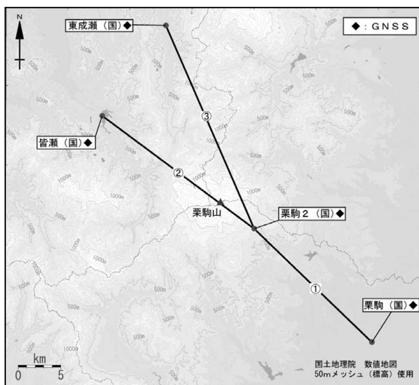
図6 栗駒山 GNSS 1) 観測点配置図
