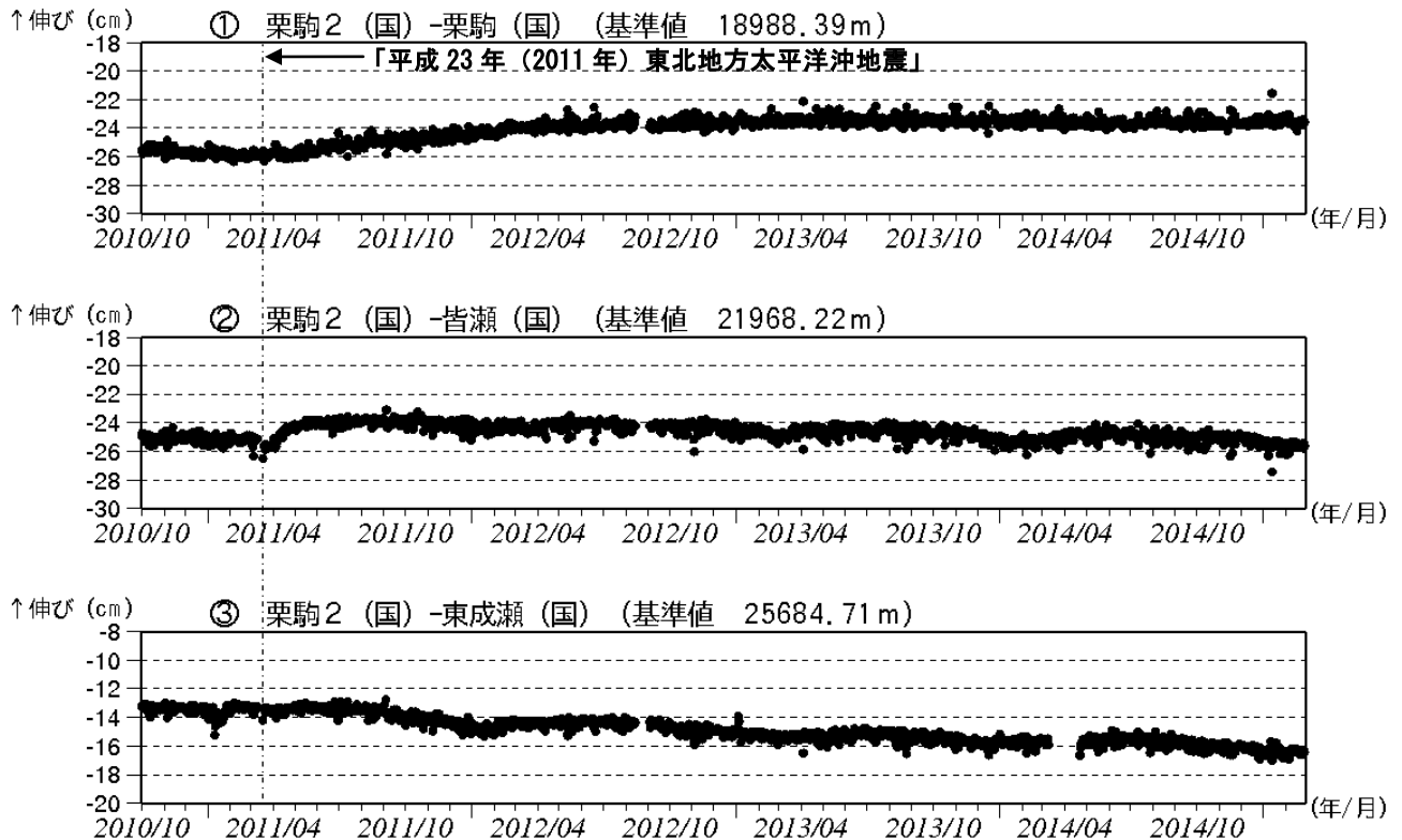
図 4 栗駒山 GNSS 基線長変化図 (2010 年 10 月～2015 年 2 月)
