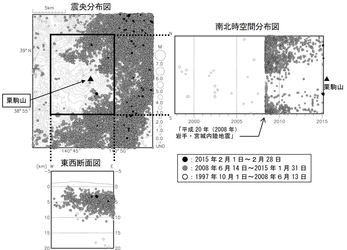
図3 栗駒山 広域地震観測網による栗駒山周辺の地震活動 (1997年10月～2015年2月)
