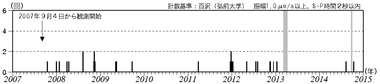
図2 岩木山 日別地震回数（2007年9月～2014年12月）
