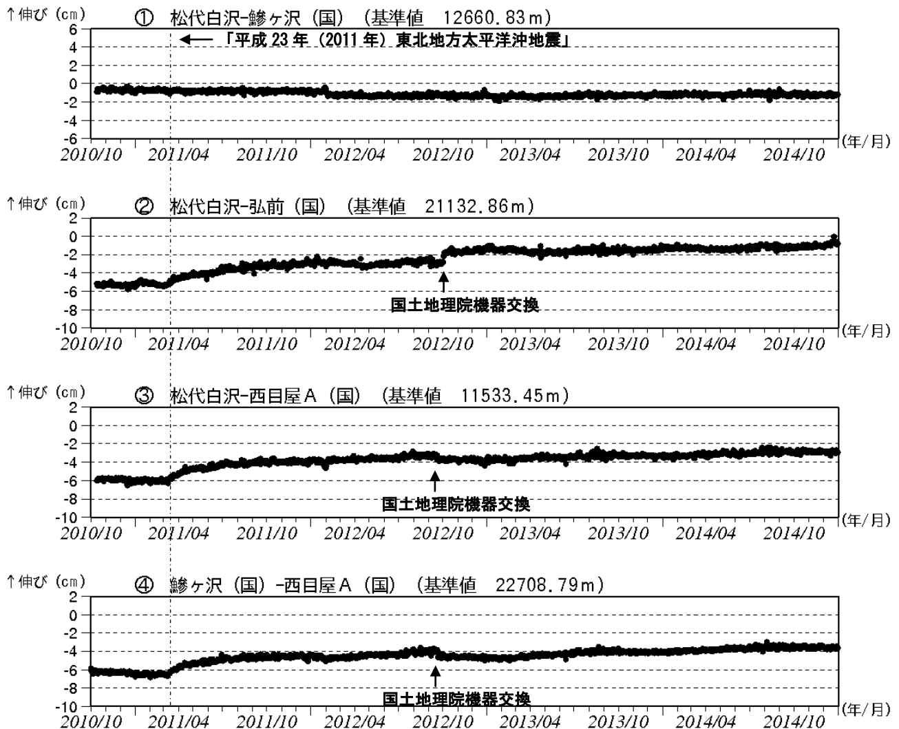
図3 岩木山 GNSS 1) 基線長変化図（2010年10月～2014年12月）
