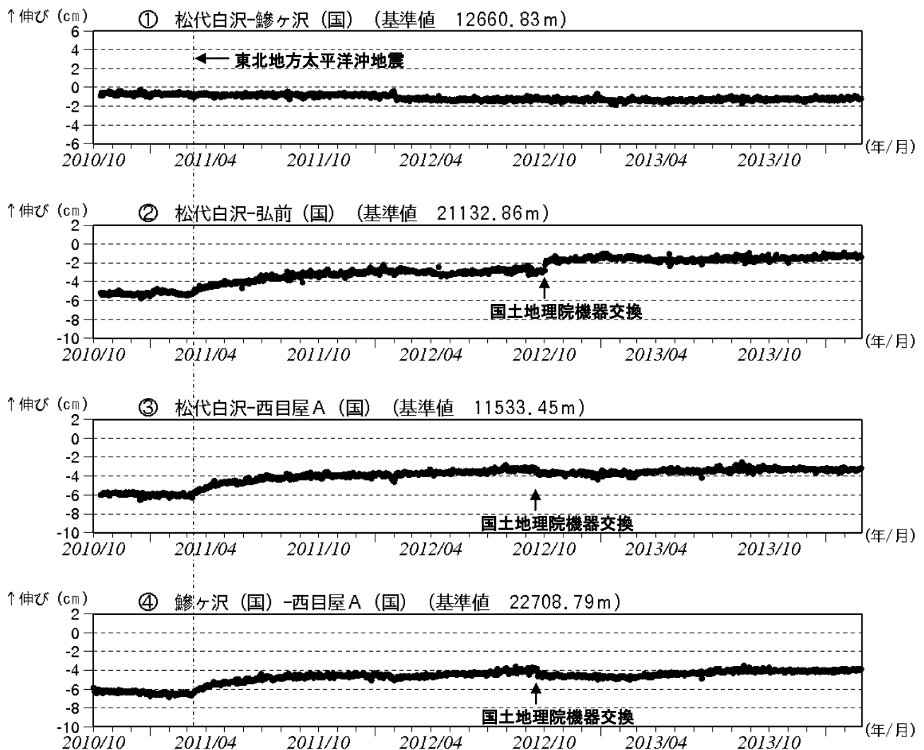
図3 岩木山 GNSS 基線長変化図（2010年10月～2014年2月）
