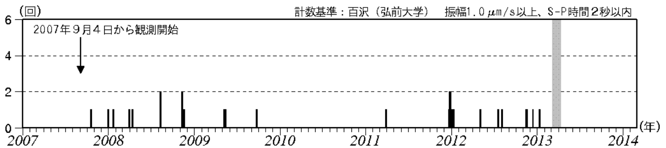
図2 岩木山 日別地震回数（2007年9月～2014年2月）
