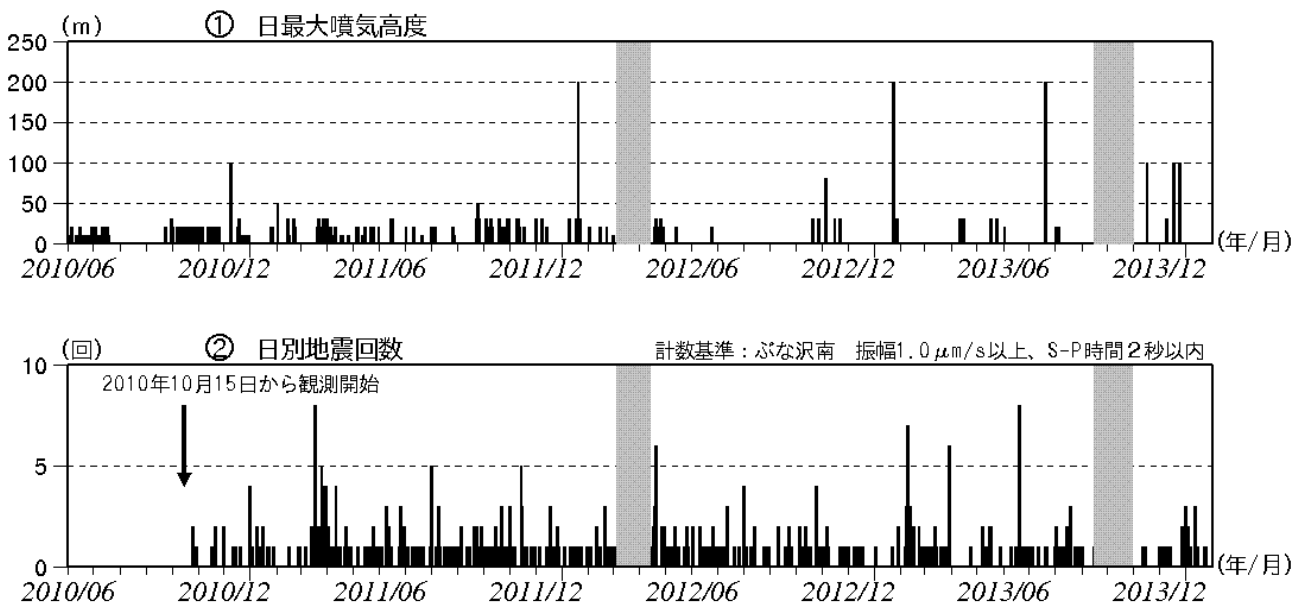
図 2 秋田焼山 火山活動経過図（2010 年 6 月～2014 年 1 月）
