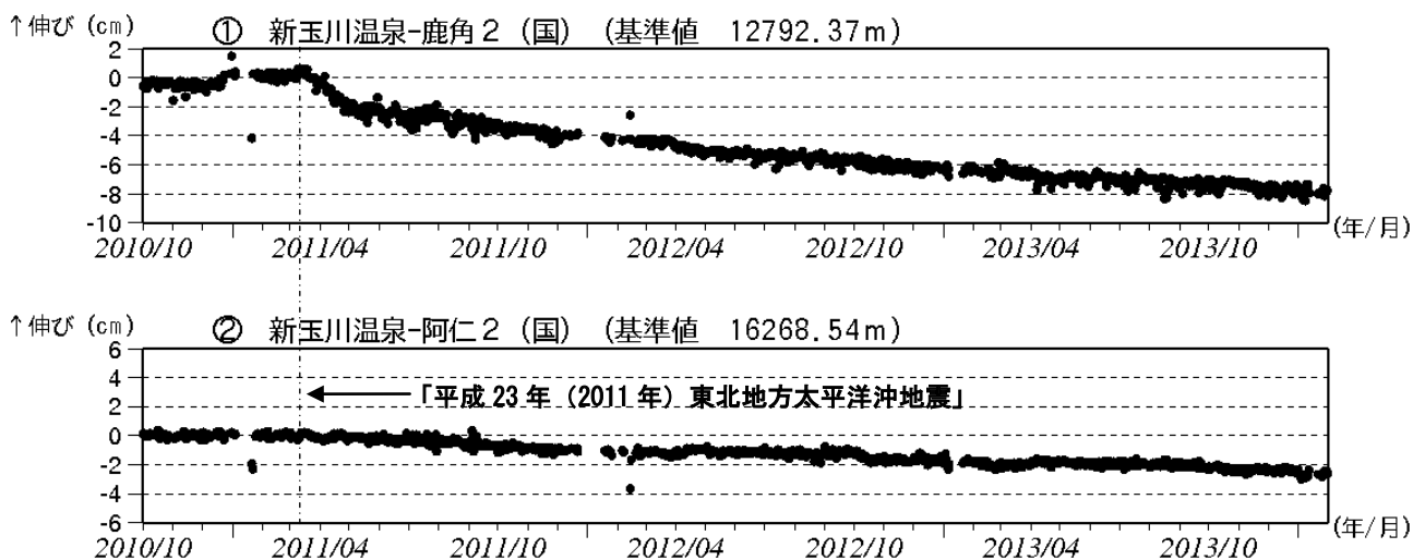
図 3 秋田焼山 GNSS 基線長変化図（2010 年 10 月～2014 年 1 月）
