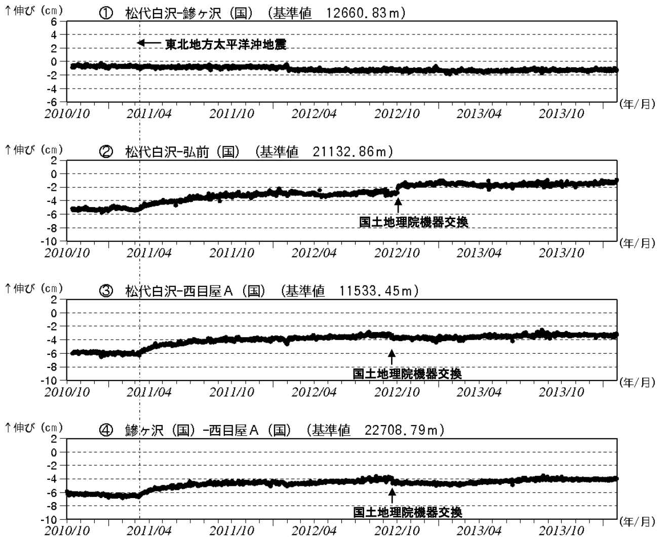
図3 岩木山 GNSS 基線長変化図（2010年10月～2014年1月）
