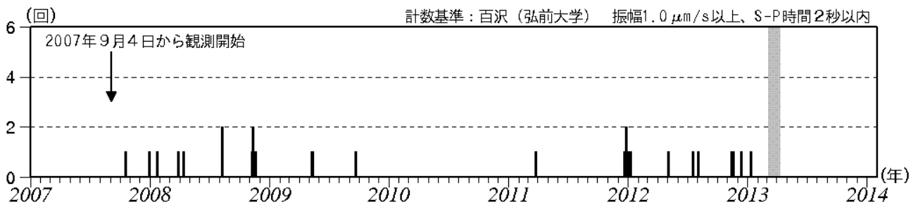
図2 岩木山 日別地震回数（2007年9月～2014年1月）
