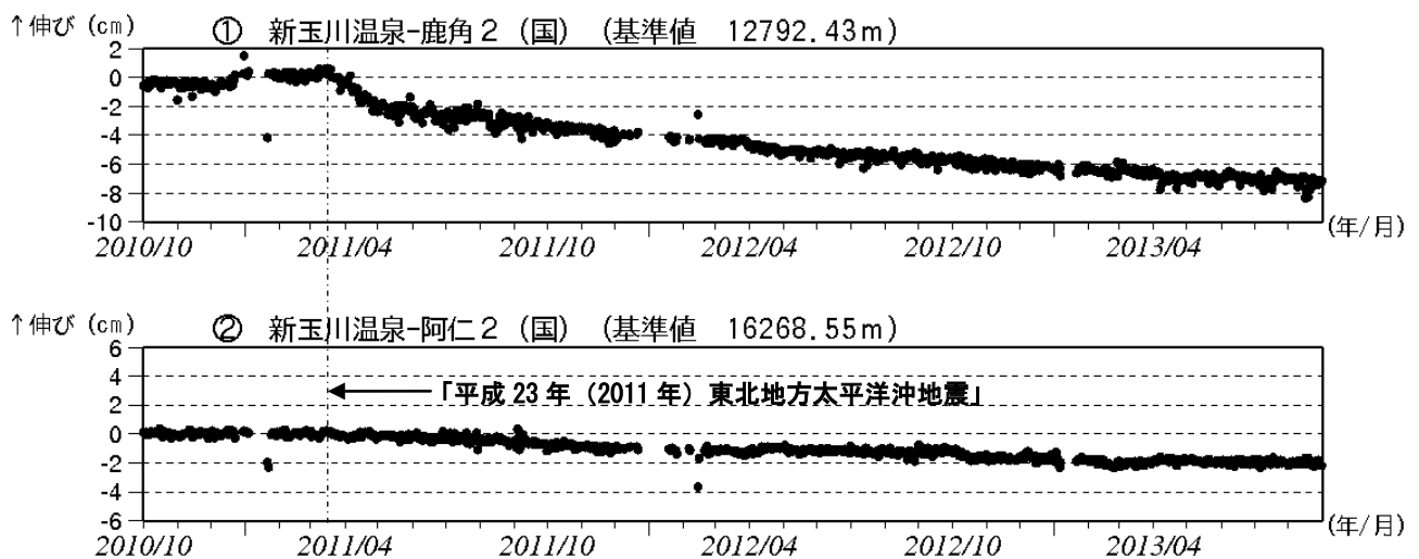
図3 秋田焼山 GPS 基線長変化図（2010年10月～2013年8月）
