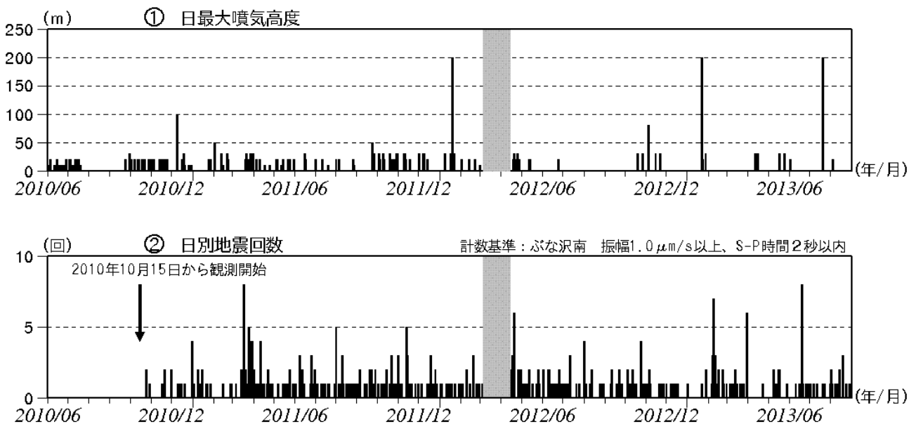
図2 秋田焼山 火山活動経過図（2010年6月～2013年8月）
