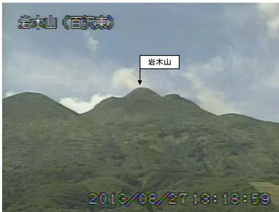
図 1 岩木山 山頂部の状況（8 月 27 日 13 時 19 分頃）
