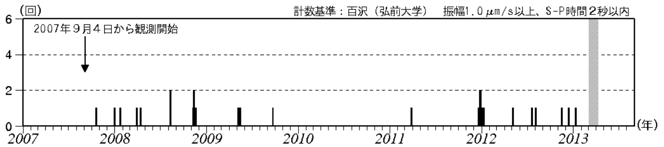
図2 岩木山 日別地震回数（2007年9月～2013年8月）
