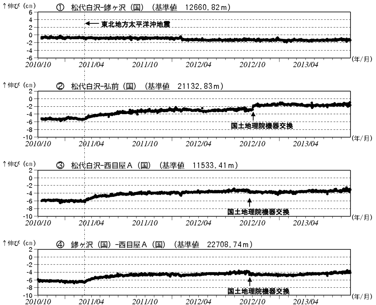
図3 岩木山 GPS 基線長変化図（2010年10月～2013年8月）
