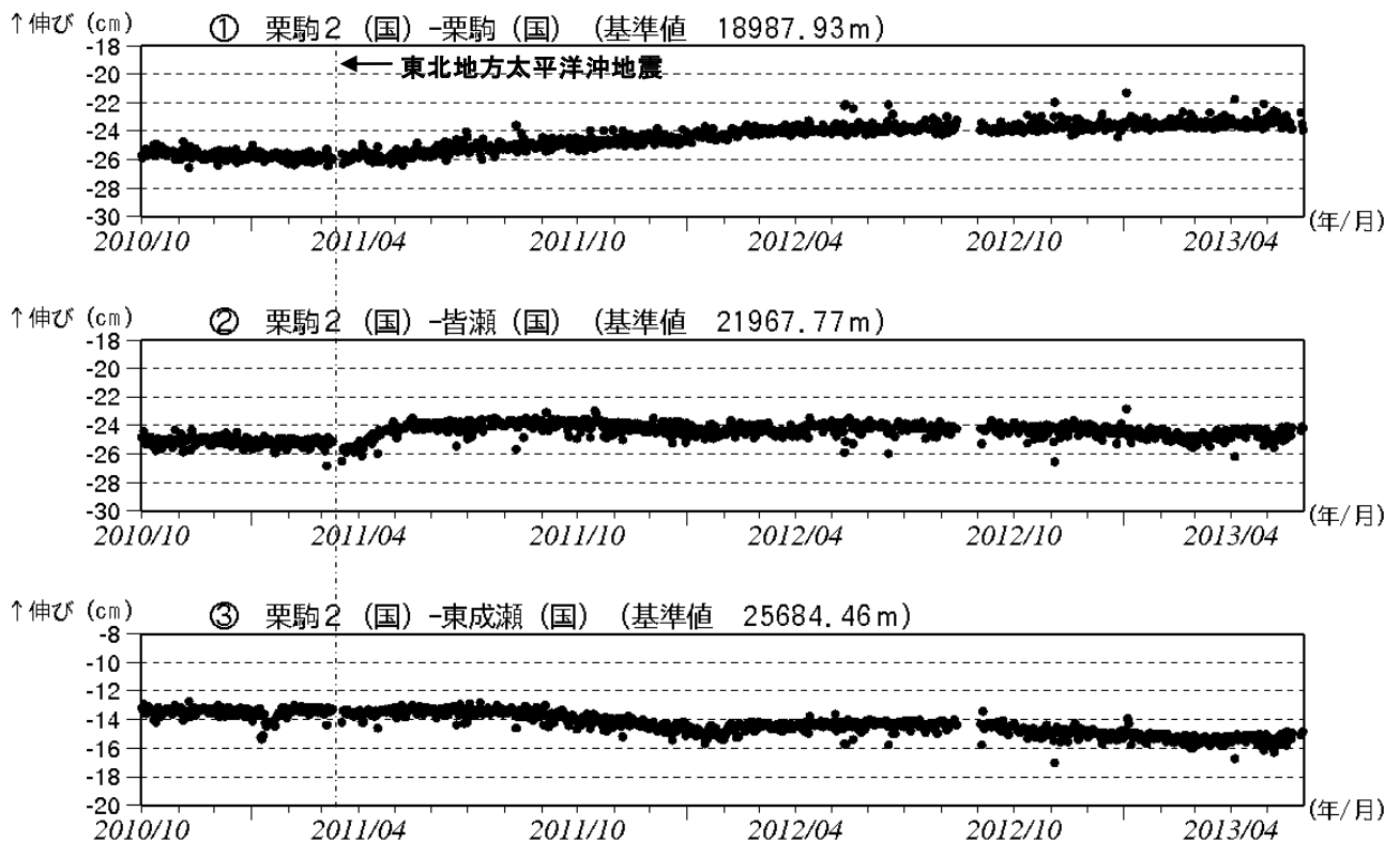
図 5 栗駒山 GPS 基線長変化図 (2010 年 10 月～2013 年 5 月)
