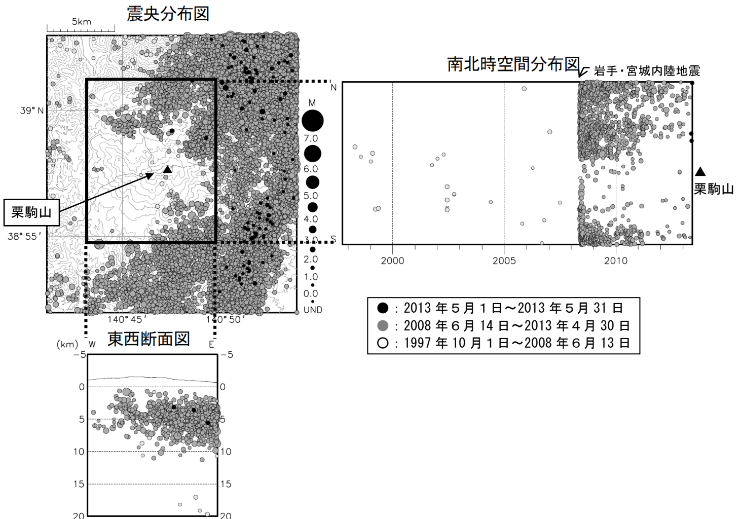
図3 栗駒山 広域地震観測網による栗駒山周辺の地震活動（1997年10月～2013年5月）
