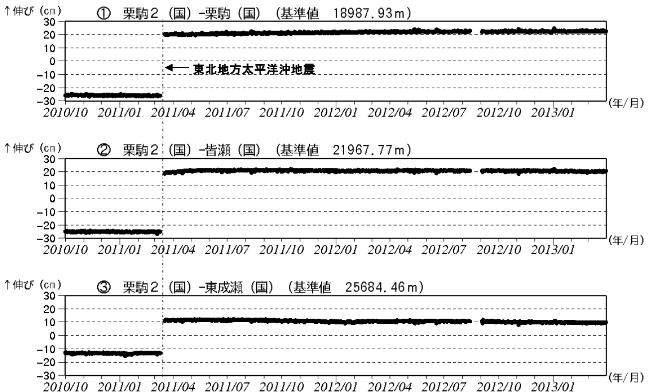
図5※ 栗駒山 GPS 基線長変化図 (2010 年 10 月～2013 年 3 月)
