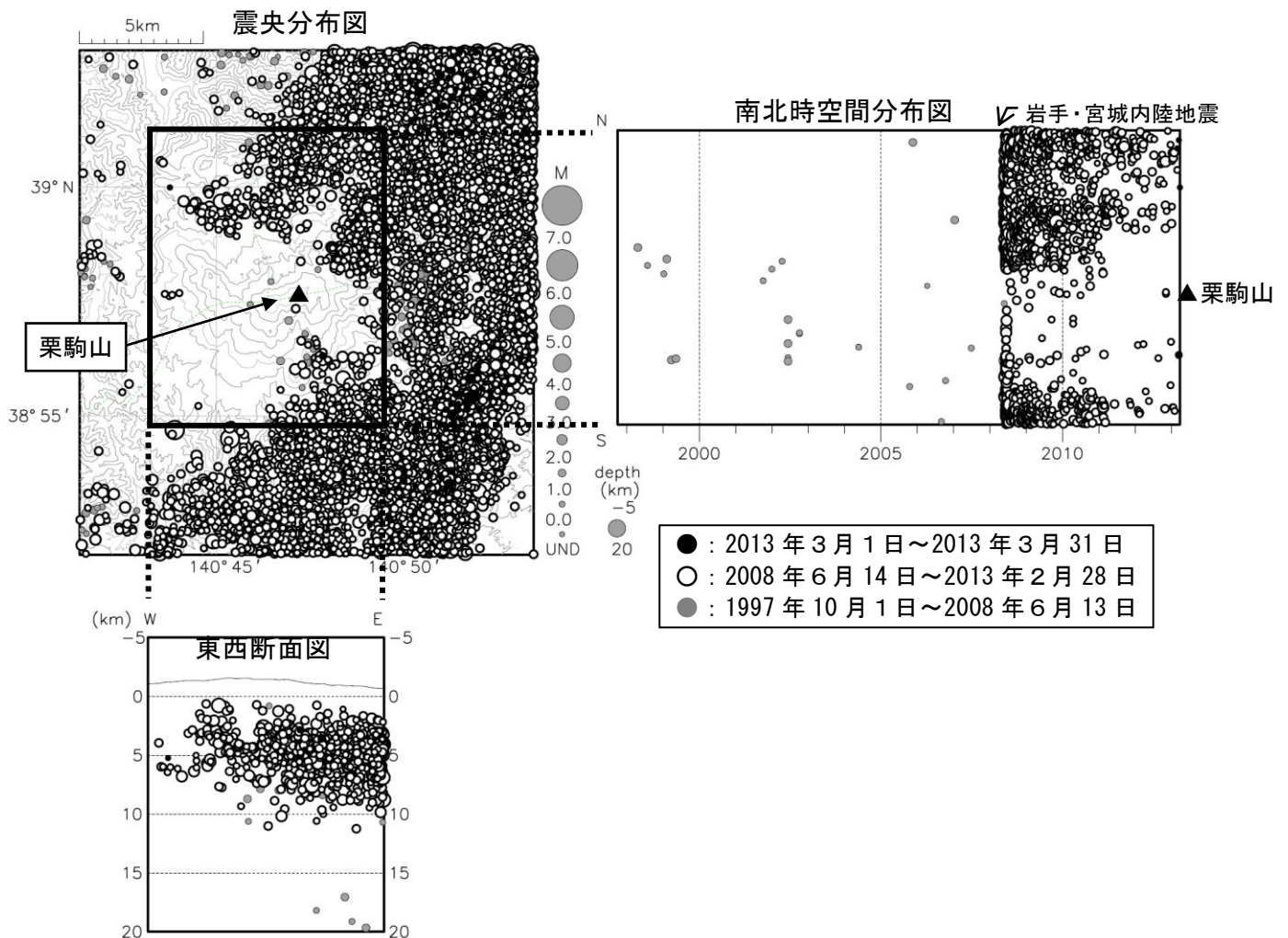
図3※ 栗駒山 広域地震観測網による栗駒山周辺の地震活動（1997年10月～2013年3月）
