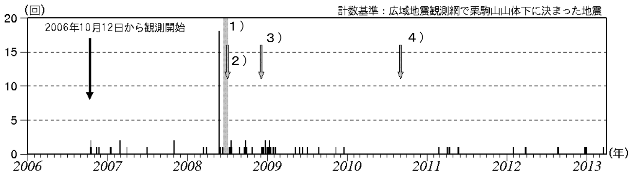
図2※ 栗駒山 日別地震回数（2006年10月～2013年3月）
