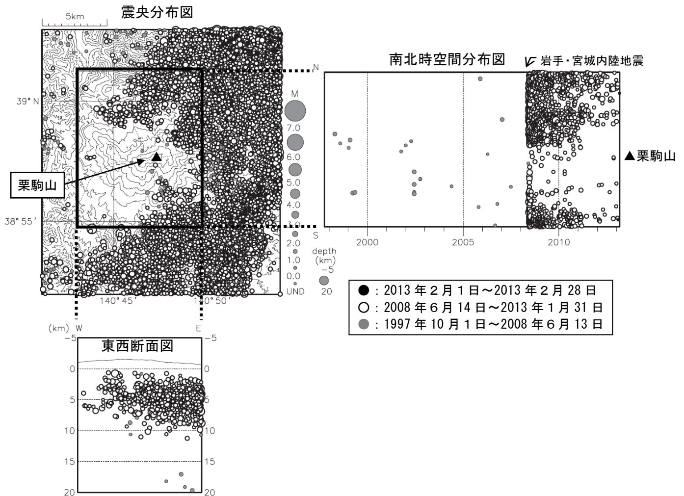
図 3※ 栗駒山 広域地震観測網による栗駒山周辺の地震活動（1997 年 10 月～2013 年 2 月）
