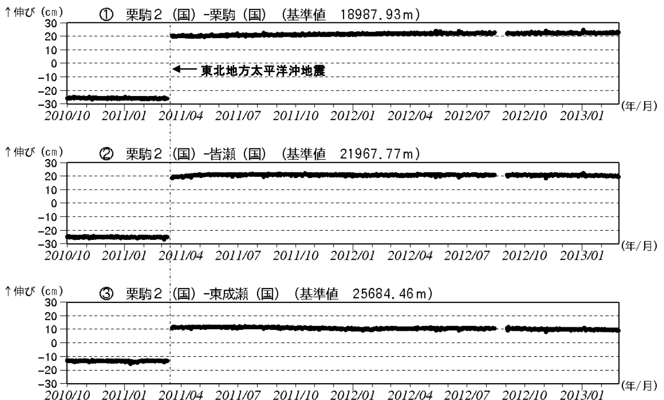
図 5＊ 栗駒山 GPS 基線長変化図 (2010 年 10 月～2013 年 2 月)
