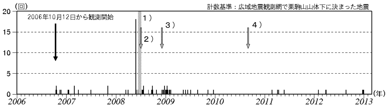
図 2※ 栗駒山 日別地震回数（2006 年 10 月～2013 年 2 月）
