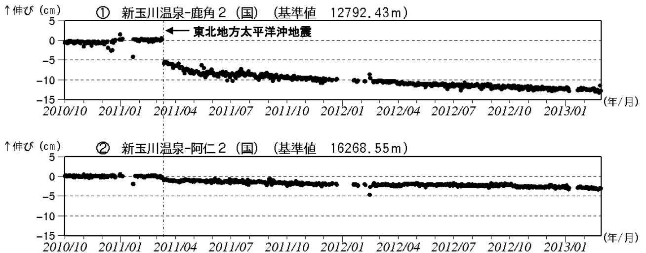
図 3* 秋田焼山 GPS 基線長変化図（2010 年 10 月～2013 年 2 月）
