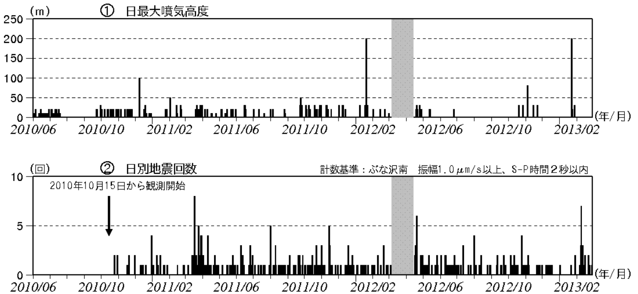
図 2 秋田焼山 火山活動経過図（2010 年 6 月～2013 年 2 月）
