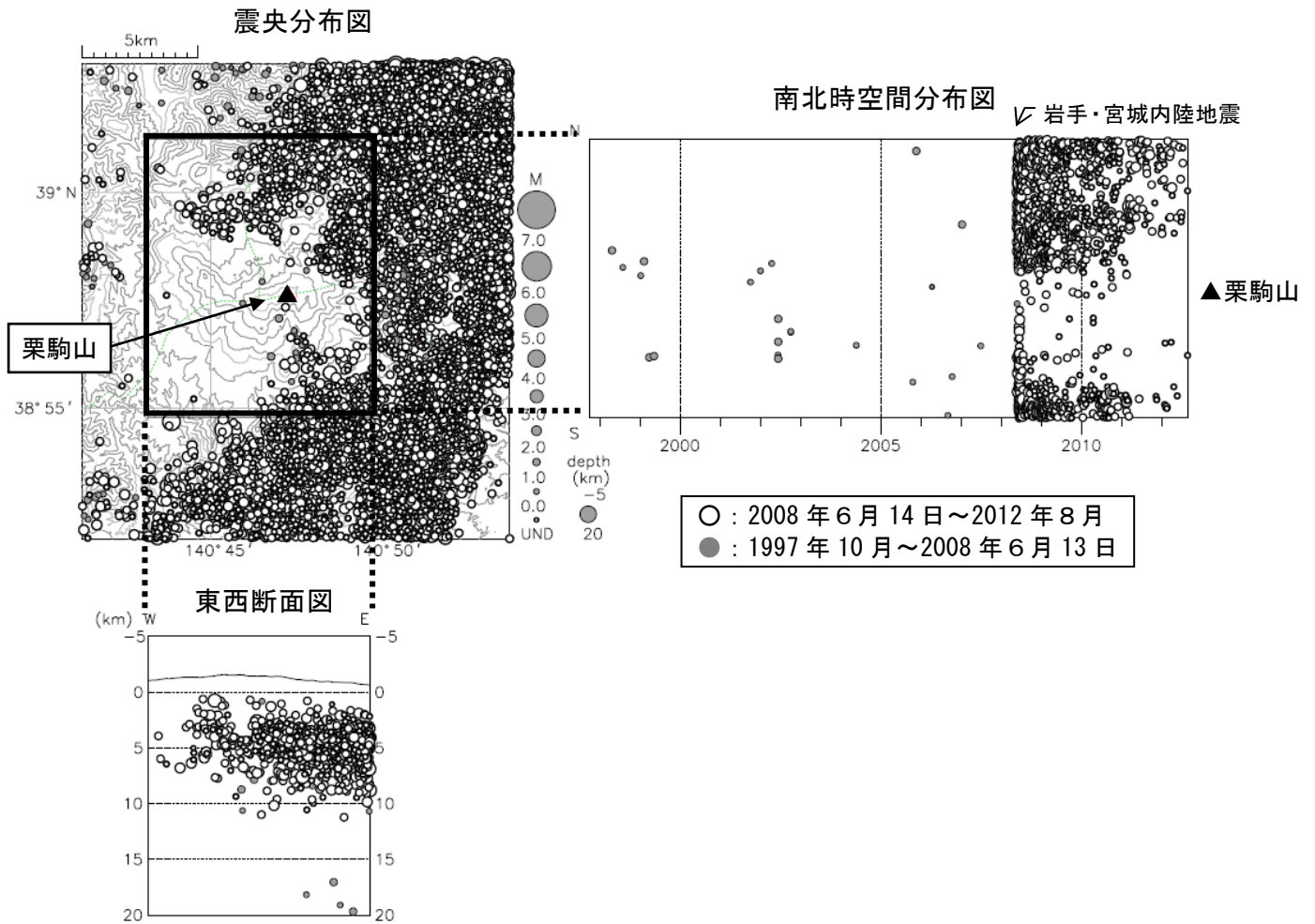
図 4※ 栗駒山 広域地震観測網による栗駒山周辺の地震活動（1997 年 10 月～2012 年 8 月）
