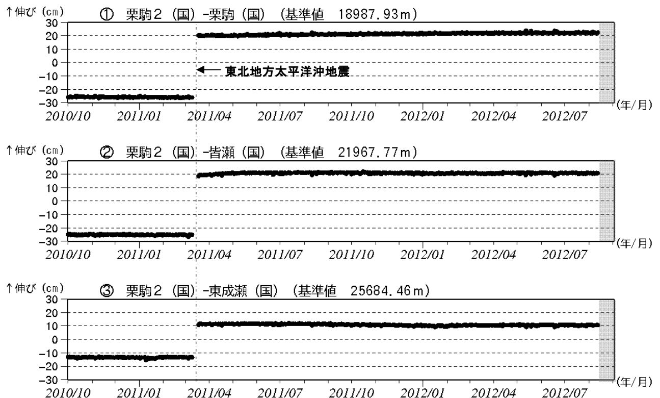
図6 栗駒山 GPS 基線長変化図（2010 年 10 月～2012 年 8 月）
