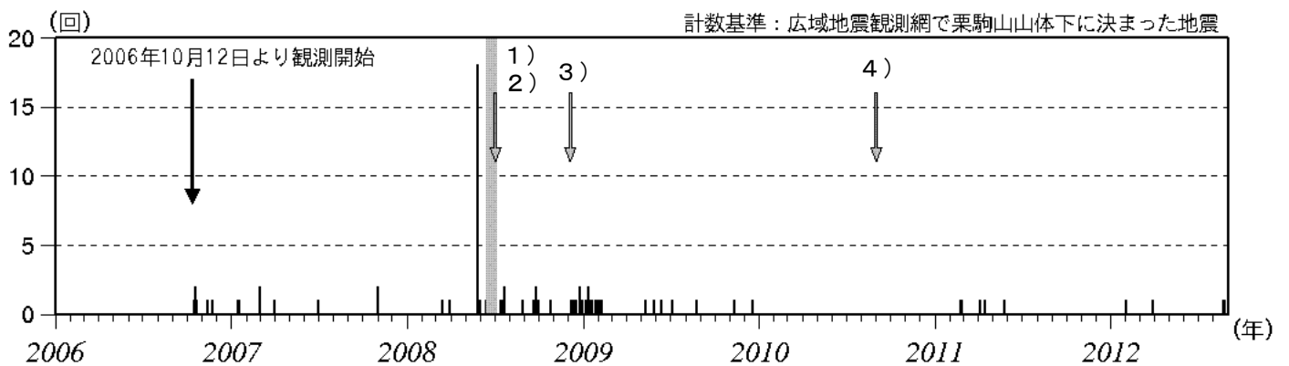
図 3※ 栗駒山 日別地震回数（2006 年 10 月～2012 年 8 月）
