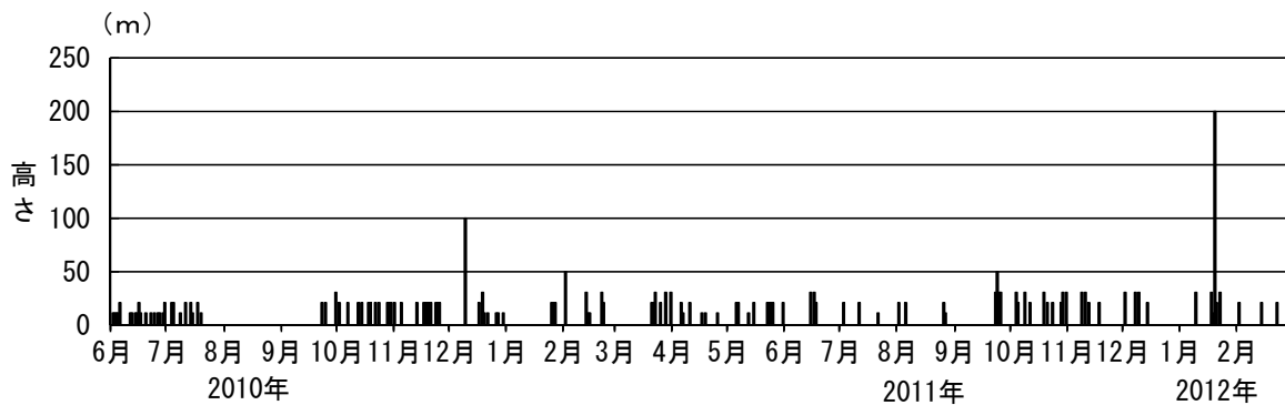
図 3※ 秋田焼山 日別最大噴気の高さ（2010 年 6 月～2012 年 2 月） 2010 年 6 月 1 日から焼山監視カメラ（東北地方整備局）により観測開始。
