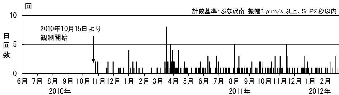
図 4 秋田焼山 火山性地震の日別回数（2010 年 10 月～2012 年 2 月） 2010 年 10 月 15 日から観測開始。
