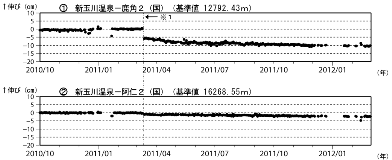
図 6※ 秋田焼山 GPS 基線長変化図（2010 年 10 月～2012 年 2 月）
