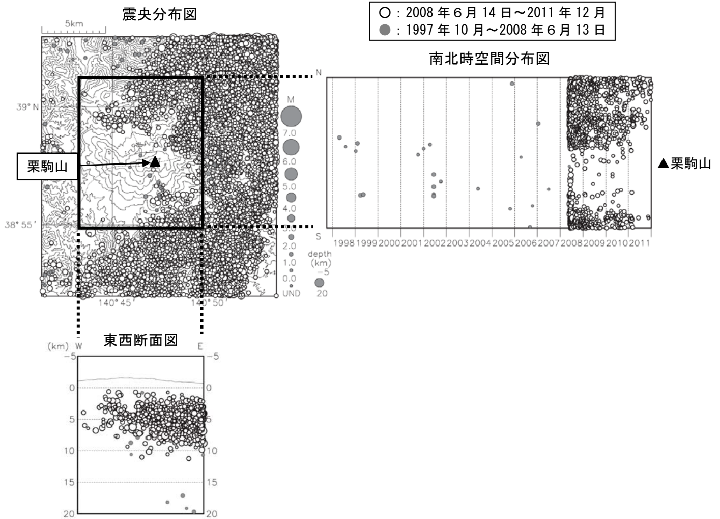
図 4 ※ 広域地震観測網による栗駒山周辺の地震活動（1997 年 10 月～2011 年 12 月）
