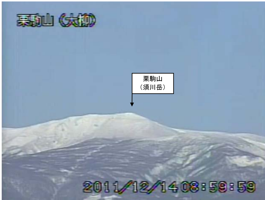
図 2 栗駒山 遠望カメラの映像（12 月 14 日 09 時 00 分頃） 大柳（山頂の南東約 20km）に設置してある遠望カメラによる。
