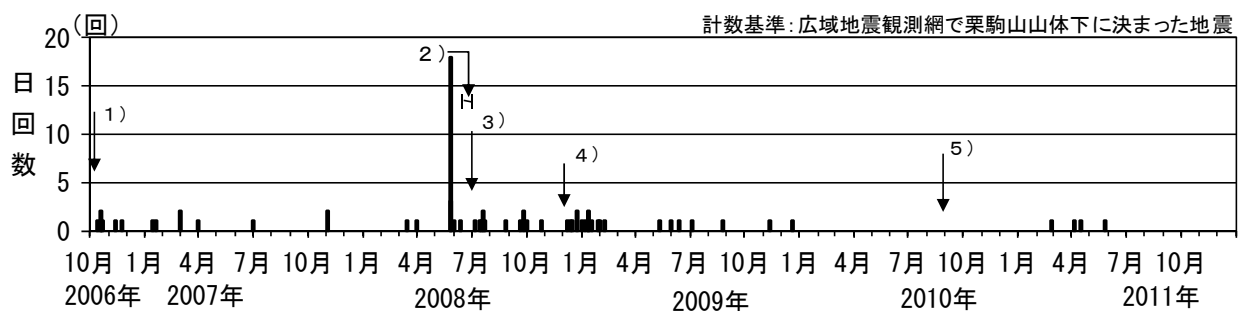
図 3※ 栗駒山 日別地震回数（2006 年 10 月～2011 年 12 月）
