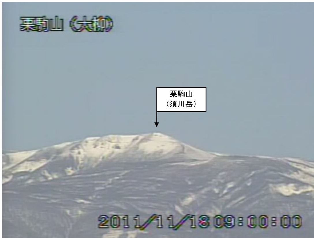
図2 栗駒山 遠望カメラの映像（11月18日09時00分頃） 大柳（山頂の南東約20km）に設置してある遠望カメラによる。
