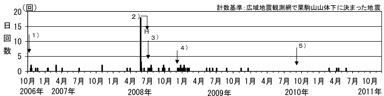
図3※ 栗駒山 日別地震回数（2006年10月～2011年11月）
