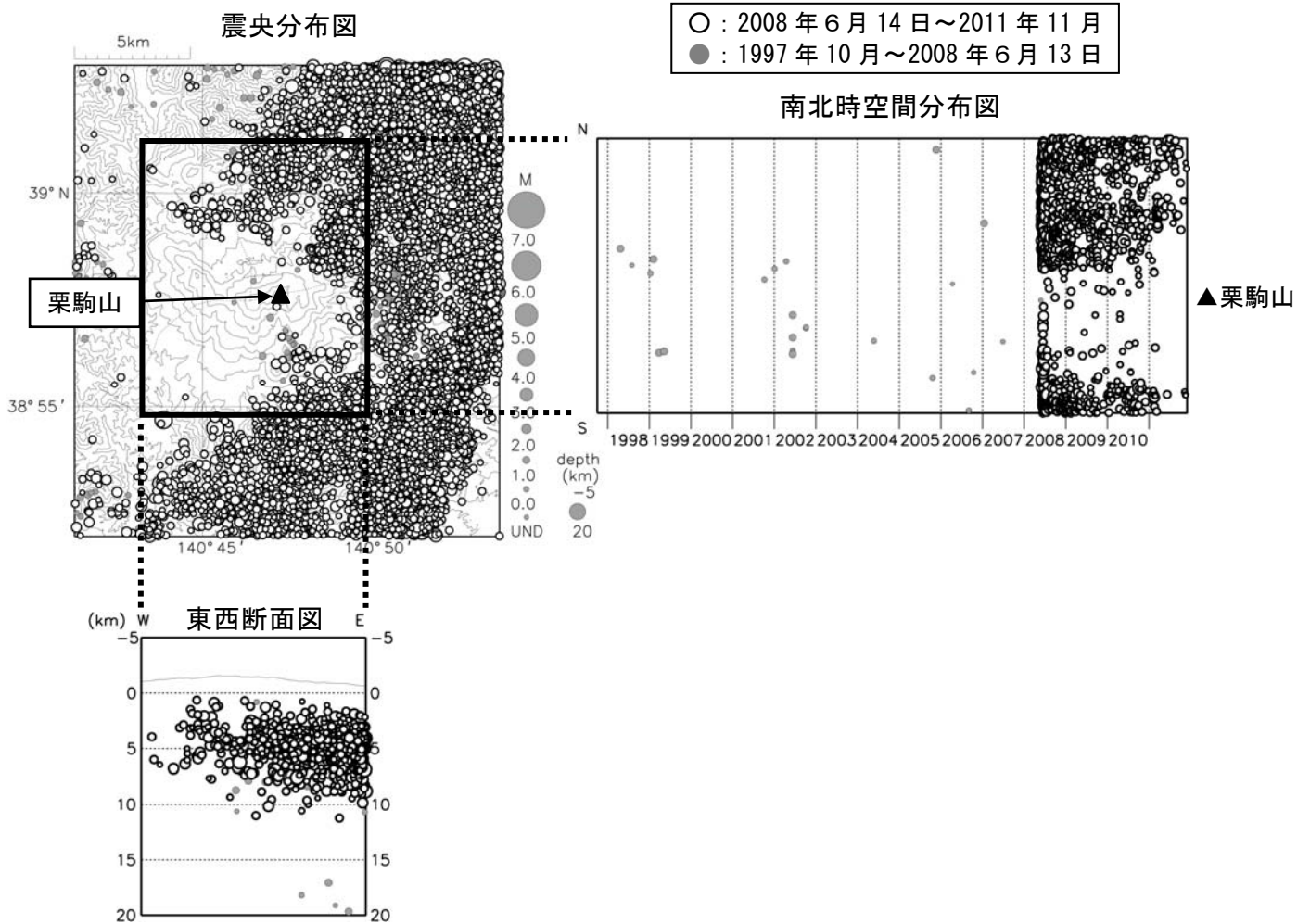
図 4 ※ 広域地震観測網による栗駒山周辺の地震活動（1997 年 10 月～2011 年 11 月）
