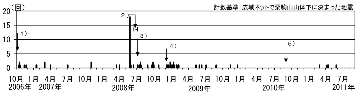
図 3※ 栗駒山 日別地震回数（2006 年 10 月～2011 年 8 月）
