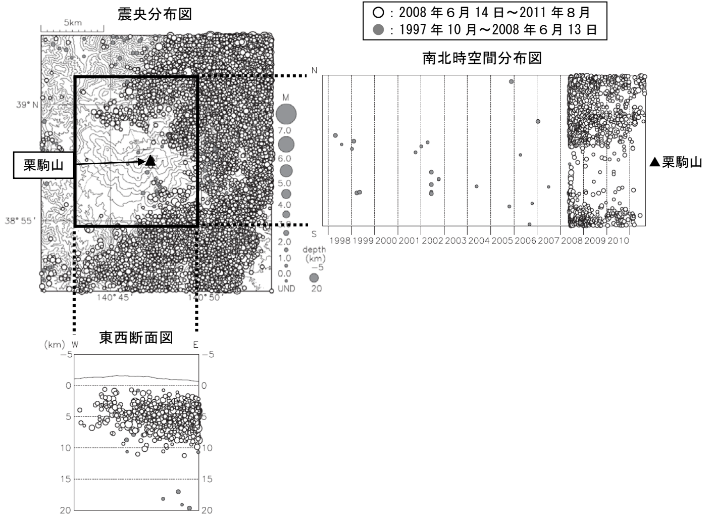
図 4 ※ 栗駒山周辺の地震活動（1997 年 10 月～2011 年 8 月）
