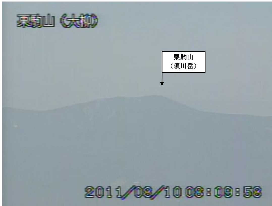
図 2 栗駒山 遠望カメラの映像（8 月 10 日 08 時 10 分頃） 大柳（山頂の南東約 20km）に設置してある遠望カメラによる。
