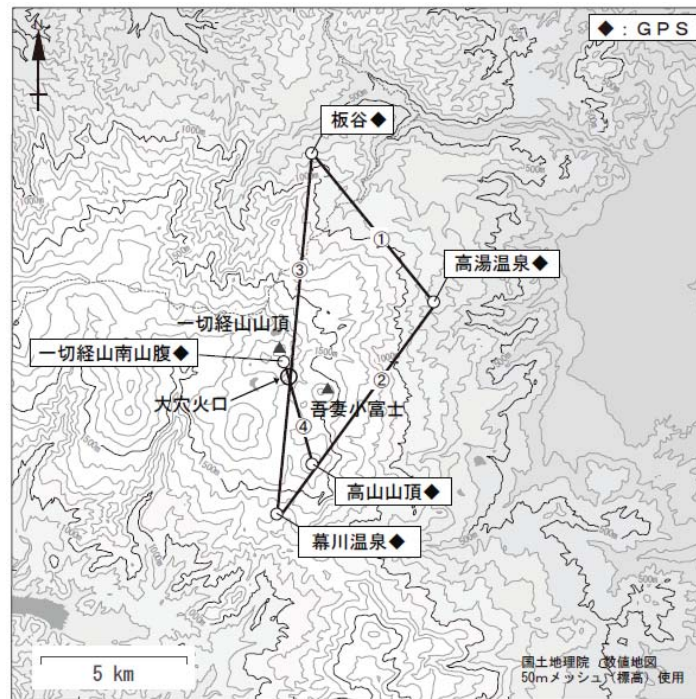
図 10 吾妻山 GPS 観測点配置図 GPS 基線①～④は図 11 の①～④に対応しています。
