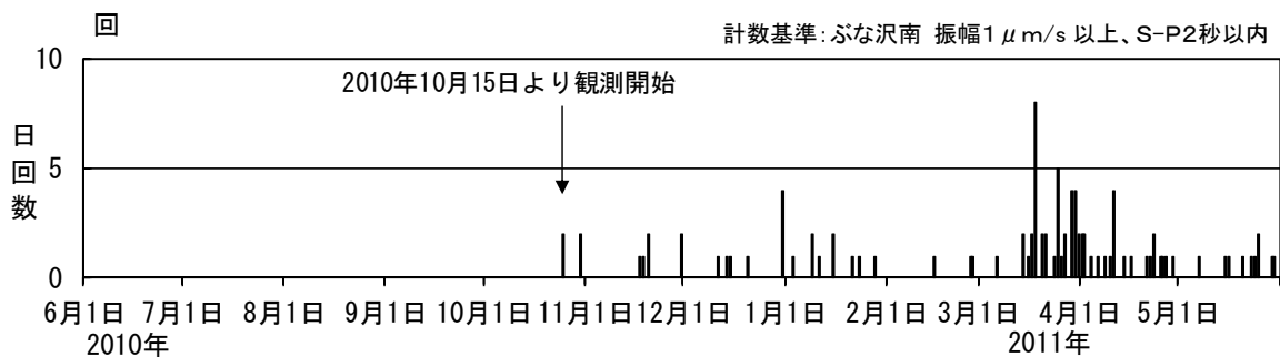
図 4 秋田焼山 火山性地震の日別回数（2010 年 10 月～2011 年 5 月）
