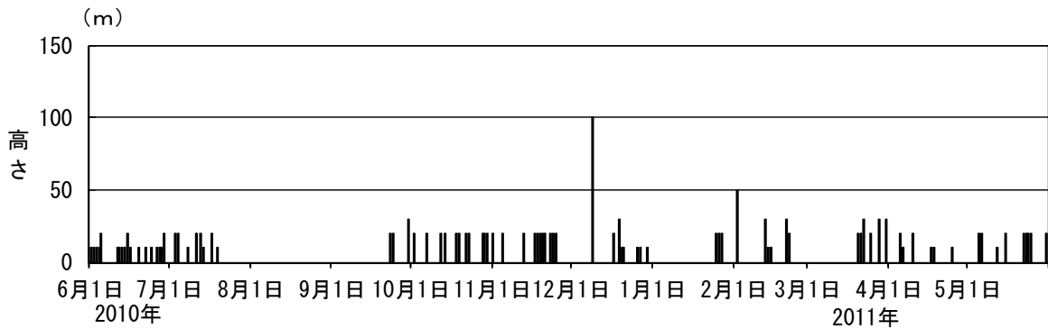
図 3※ 秋田焼山 日別最大噴気の高さ（2010 年 6 月～2011 年 5 月）
