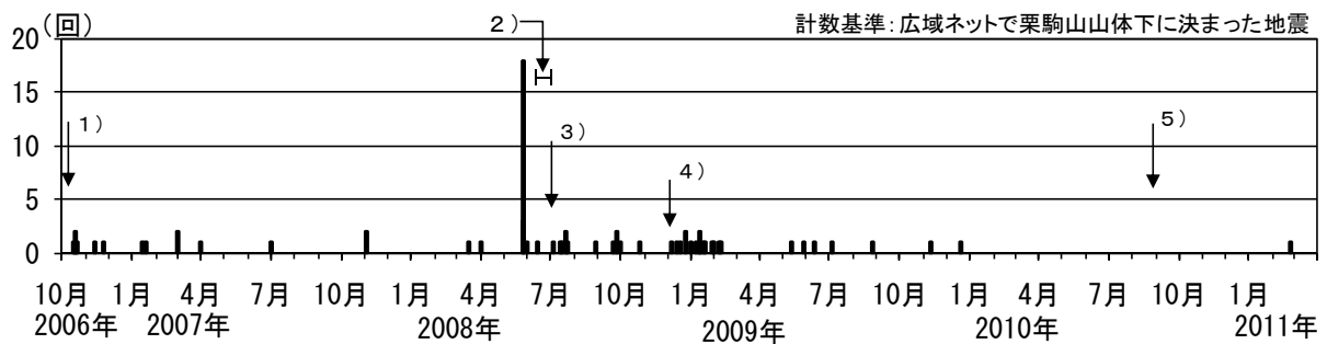
図 3※ 栗駒山 日別地震回数（2006 年 10 月～2011 年 3 月）
