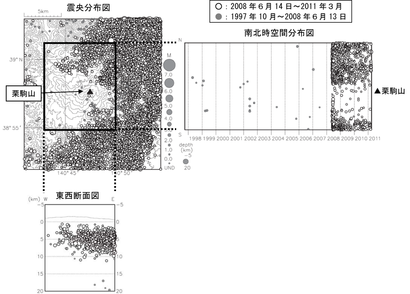
図 4※ 栗駒山周辺の地震活動（1997 年 10 月～2011 年 3 月）
