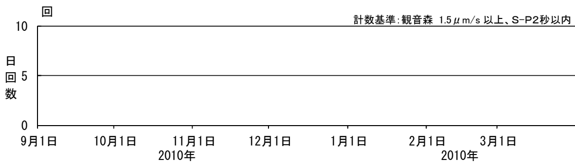
図3 鳥海山 火山性地震の日別回数（2010年9月～2011年3月）
