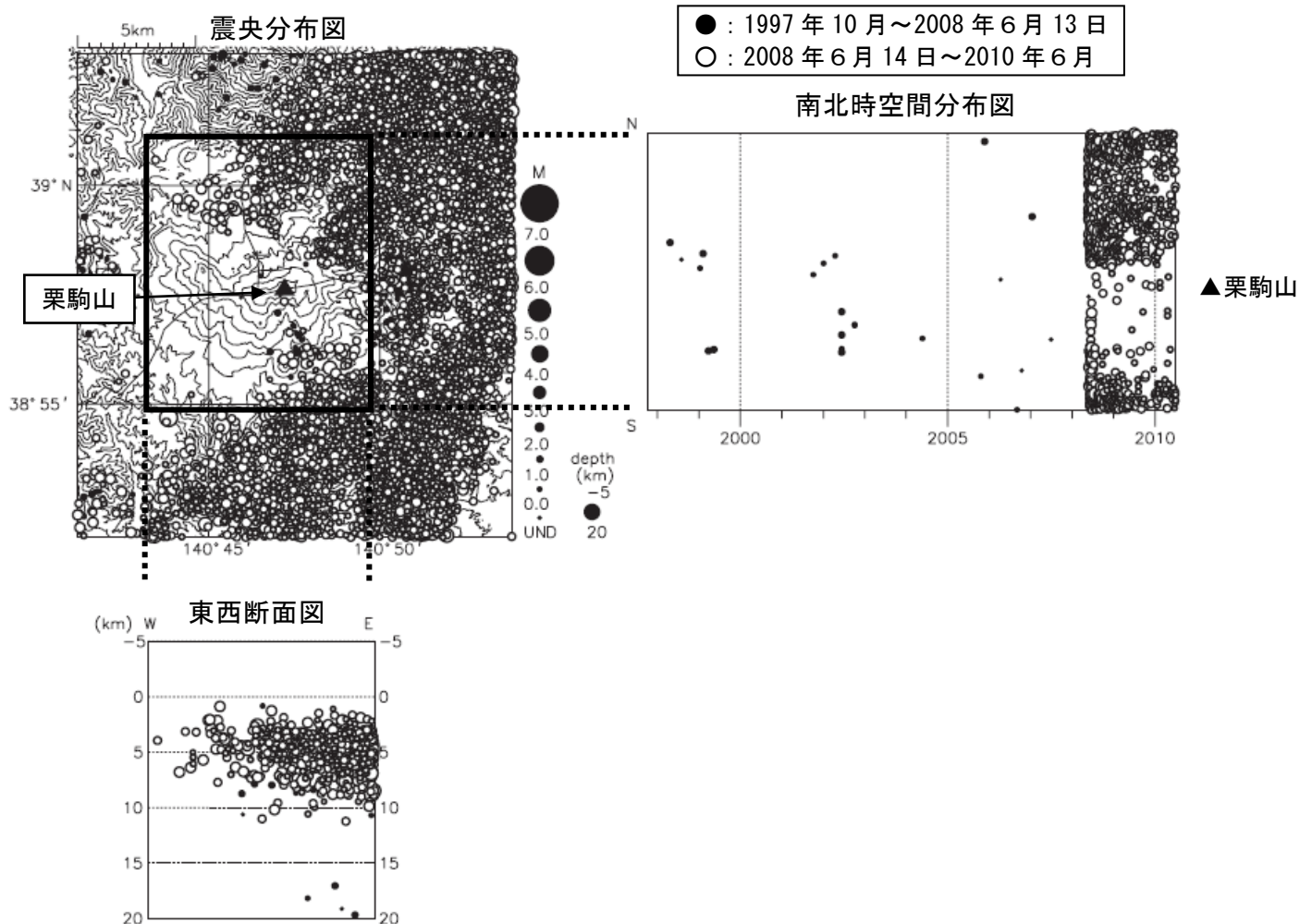
図4※ 栗駒山周辺の地震活動（1997年10月～2010年6月）
