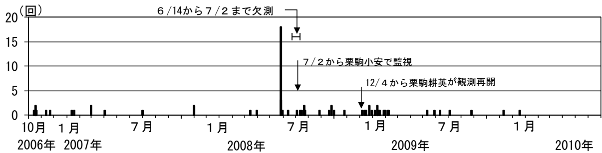
図3 栗駒山 日別地震回数（2006年10月～2010年6月）
