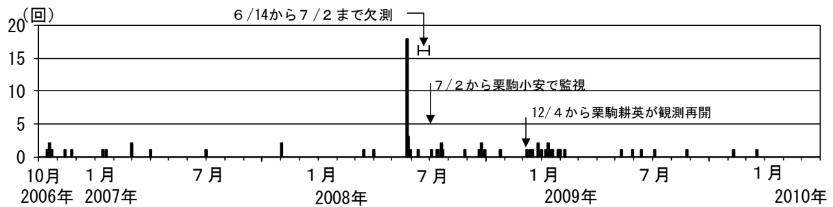
図2 栗駒山 日別地震回数（2006年10月～2010年3月）
