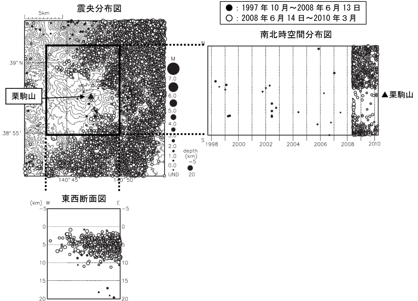
図3※ 栗駒山周辺の地震活動（1997年10月～2010年3月）
