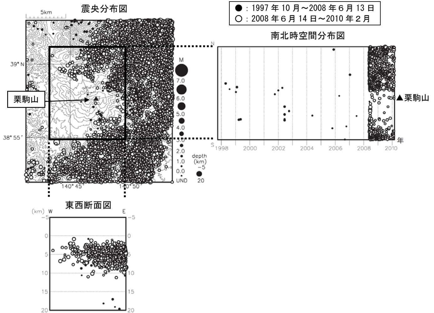
図 3※ 栗駒山周辺の地震活動（1997 年 10 月～2010 年 2 月）
