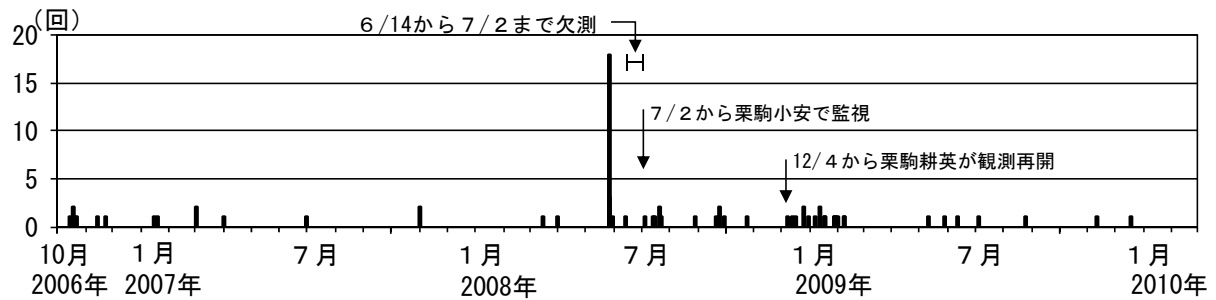
図 2 栗駒山 日別地震回数（2006 年 10 月～2010 年 2 月）
