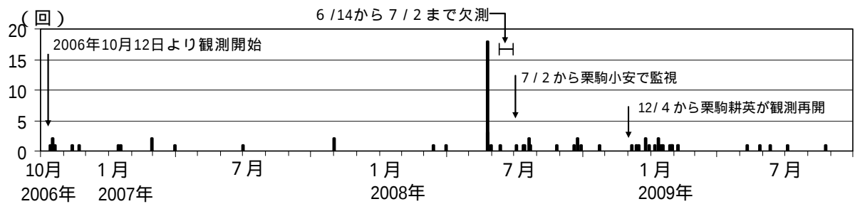
図2 栗駒山 日別地震回数（2006年10月～2009年9月）
