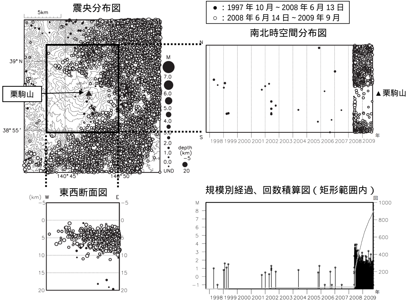
図3 栗駒山周辺の地震活動（1997年10月～2009年9月）
