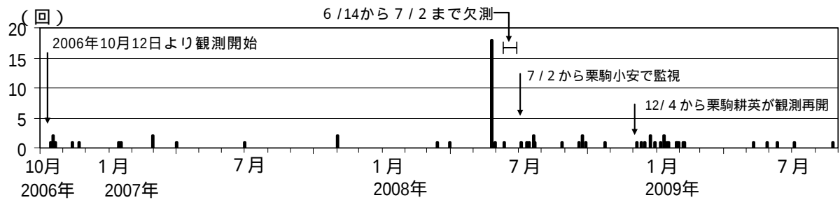
図2 栗駒山 日別地震回数（2006 年 10 月～2009 年 8 月）
