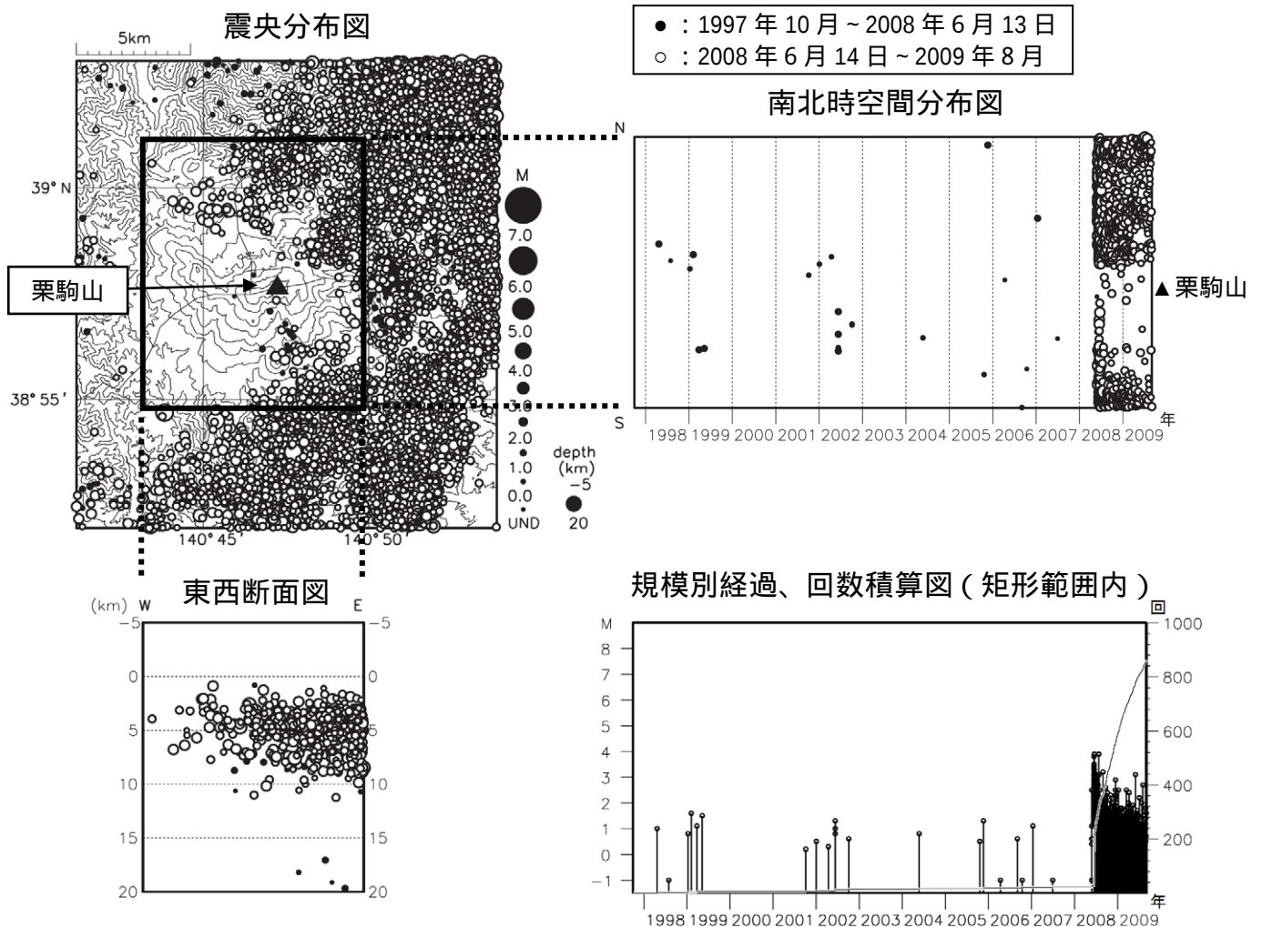
図3 栗駒山周辺の地震活動（1997 年 10 月～2009 年 8 月）
