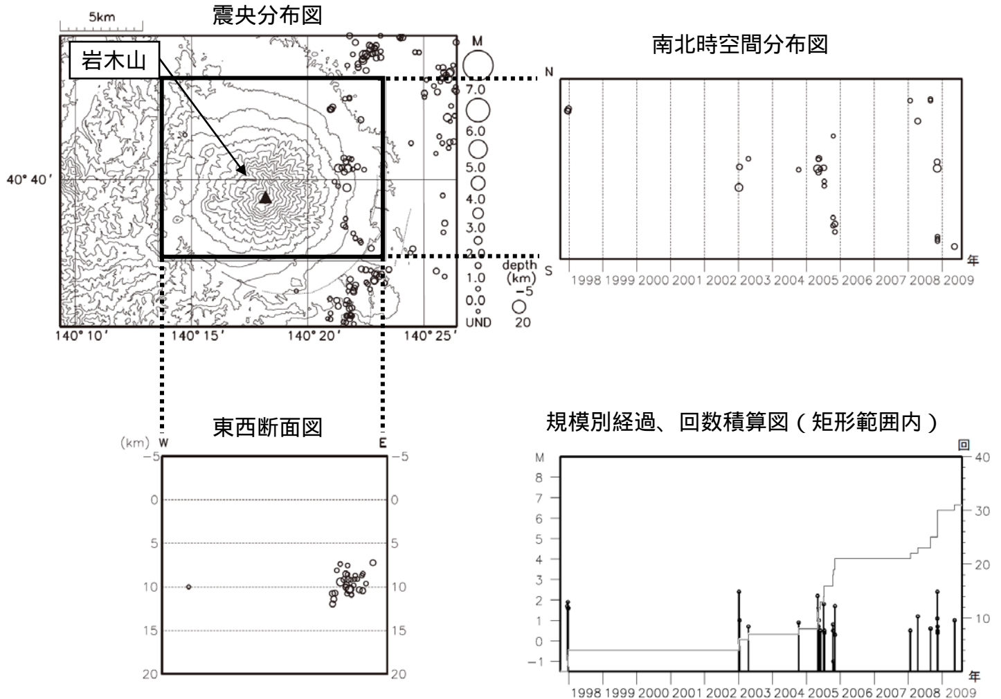
図 2 岩木山周辺の地震活動（1997 年 10 月～2009 年 7 月）
