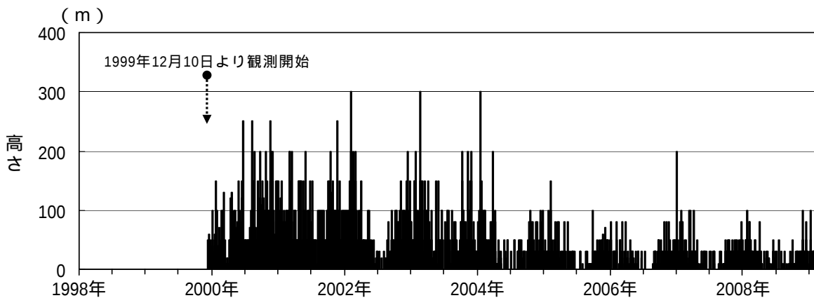
図4 岩手山 日最大噴気の高さ（黒倉山）（1999年12月10日～2009年1月）
