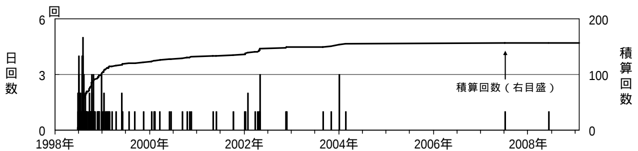
図3 岩手山 日別微動回数（1998年1月～2009年1月）
