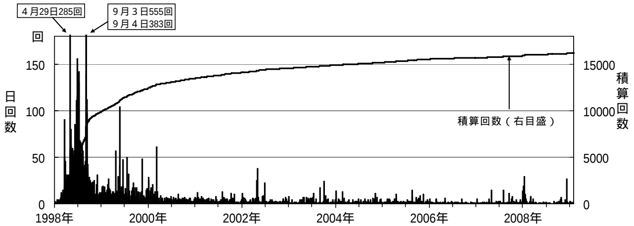
図2 岩手山 日別地震回数（1998年1月～2009年1月）
