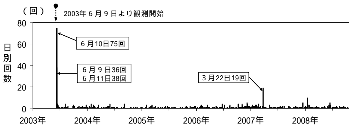
図 2 秋田駒ヶ岳 日別地震回数（2003 年 6 月 9 日～2008 年 11 月）
