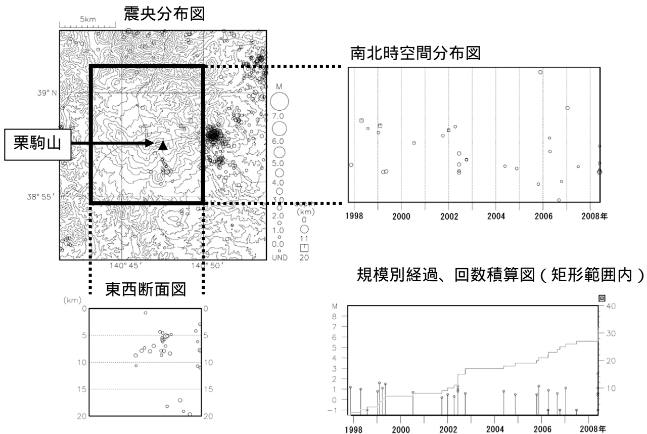
図 3 栗駒山周辺の地震活動（1997 年 10 月～2008 年 5 月）
