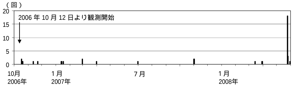
図 2 栗駒山 日別地震回数（2006 年 10 月～2008 年 5 月）
