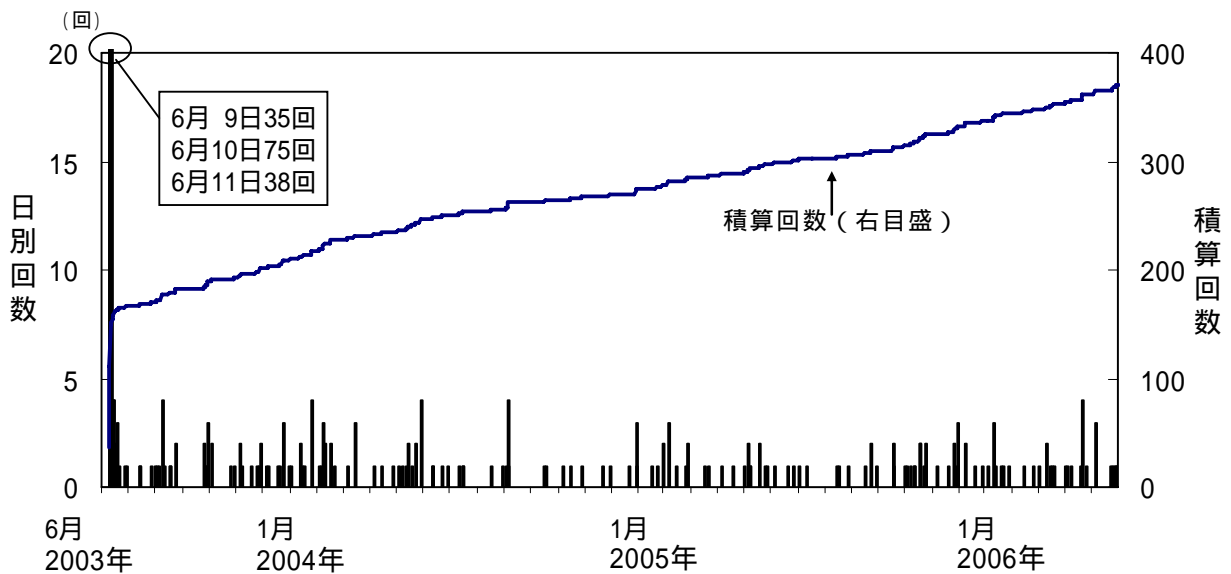
図2 秋田駒ヶ岳 日別地震回数（2003年6月9日～2006年7月）
