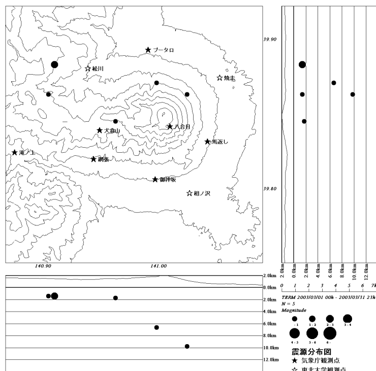
岩手山震源分布図 (2003.03.01 ~ 03.31)
