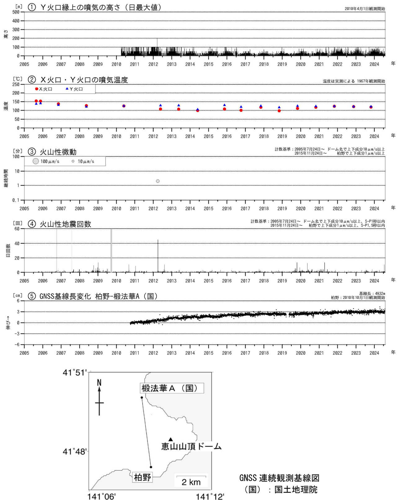
図2 恵山 火山活動経過図（2005年7月～2024年7月） ④の灰色部分は機器障害による欠測期間を示します。 ⑤のグラフは上図の基線に対応しています。 ⑤のグラフの空白部分は欠測を示します。
