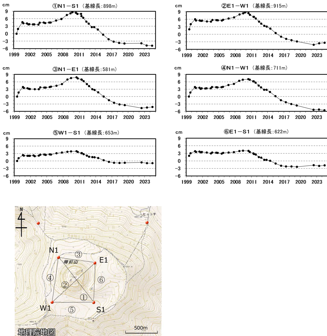
図4 樽前山 GNSS 繰り返し観測による基線長変化（1999 年 7 月～2024 年 6 月）及び観測点配置図と基線組み合わせ ・ 6 月 6 ～10 日に実施した繰り返し観測の結果、前回（2023 年 6 月）の観測と比べて特段の変化は認められませんでした。
