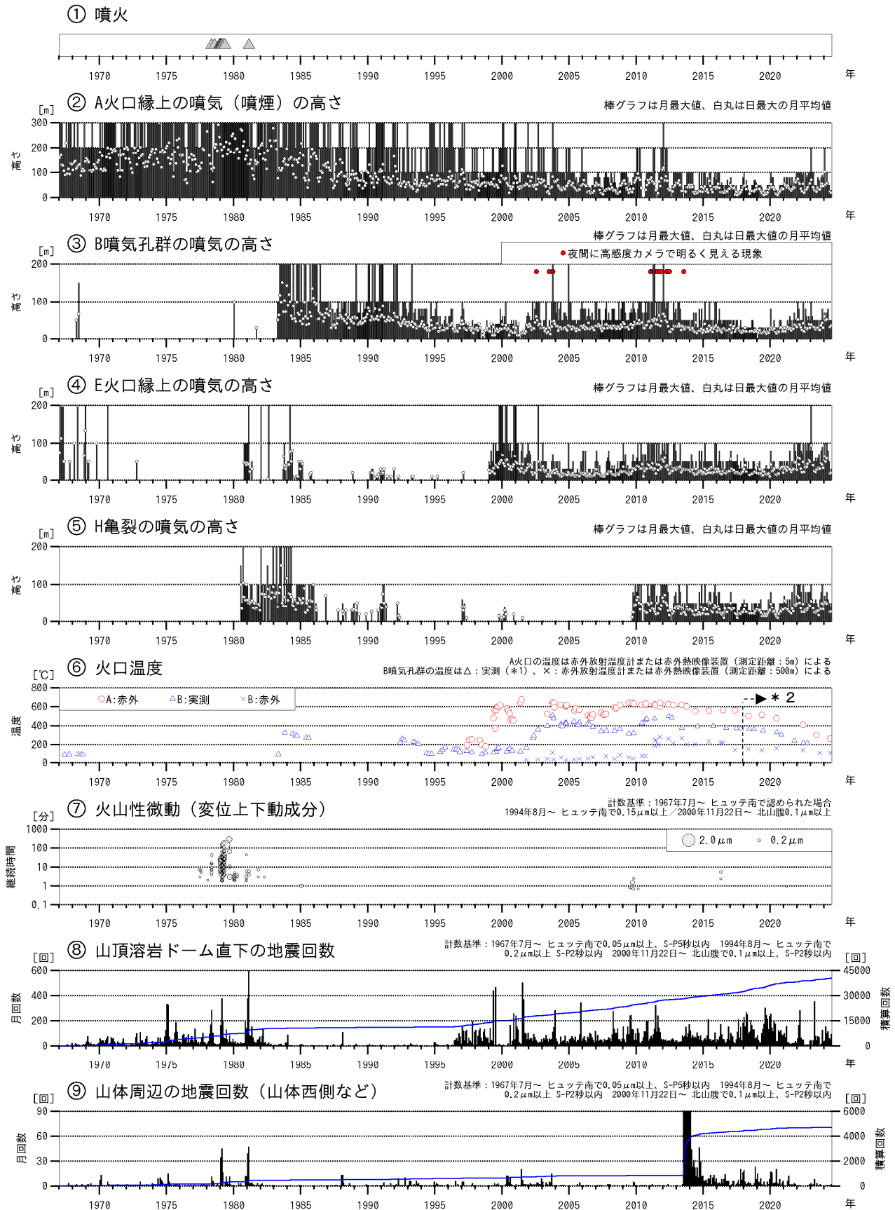
図2 樽前山 火山活動経過図（1967年1月～2024年7月）
