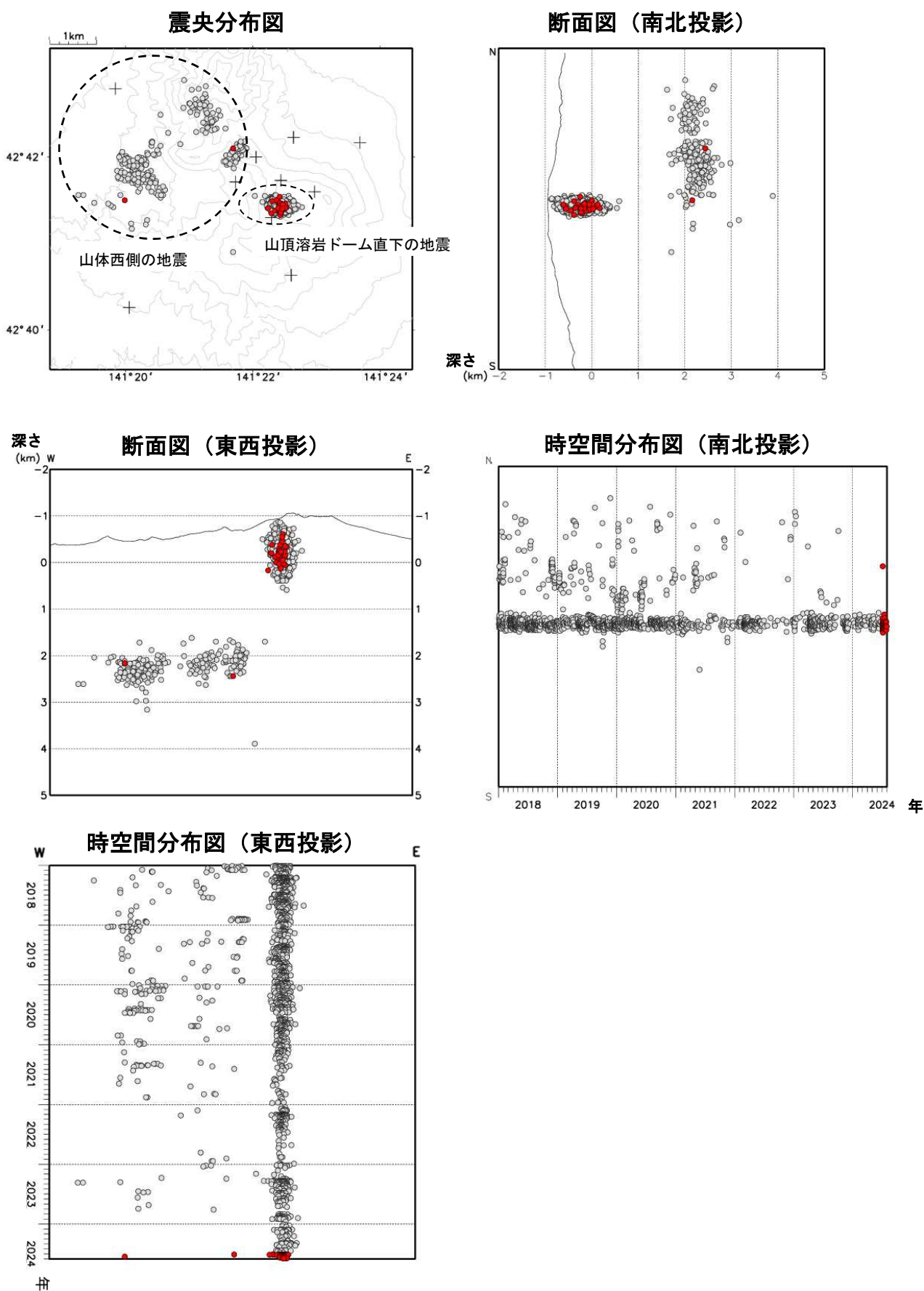
図3 樽前山 火山性地震の震源分布（2018年1月～2024年7月）
