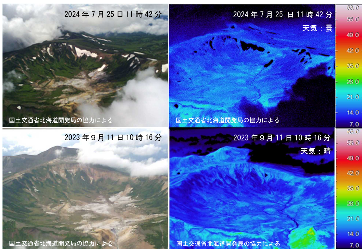
図5 大雪山 赤外熱映像観測装置による御鉢平の地表面温度分布
