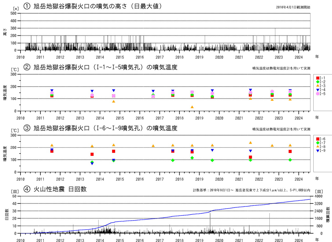
図2 大雪山 火山活動経過図（2010年4月～2024年7月）
