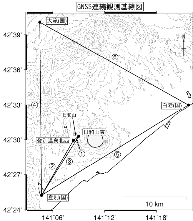
図10 倶多楽 観測点配置図
