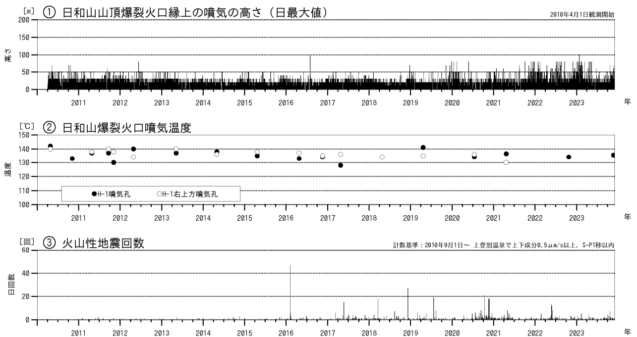
図2 倶多楽 火山活動経過図（2010年1月～2023年11月）
