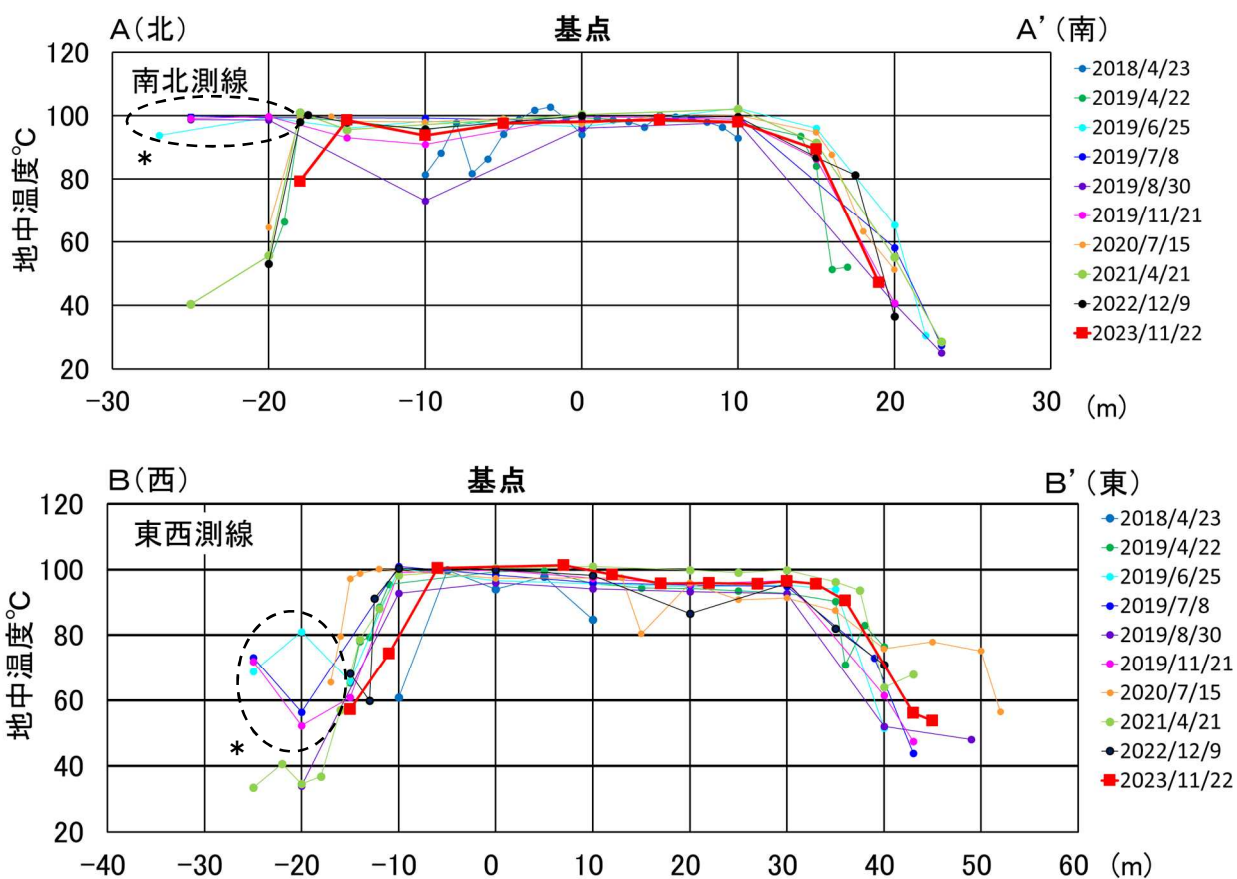
図8 倶多楽 笠山の地中温度分布
