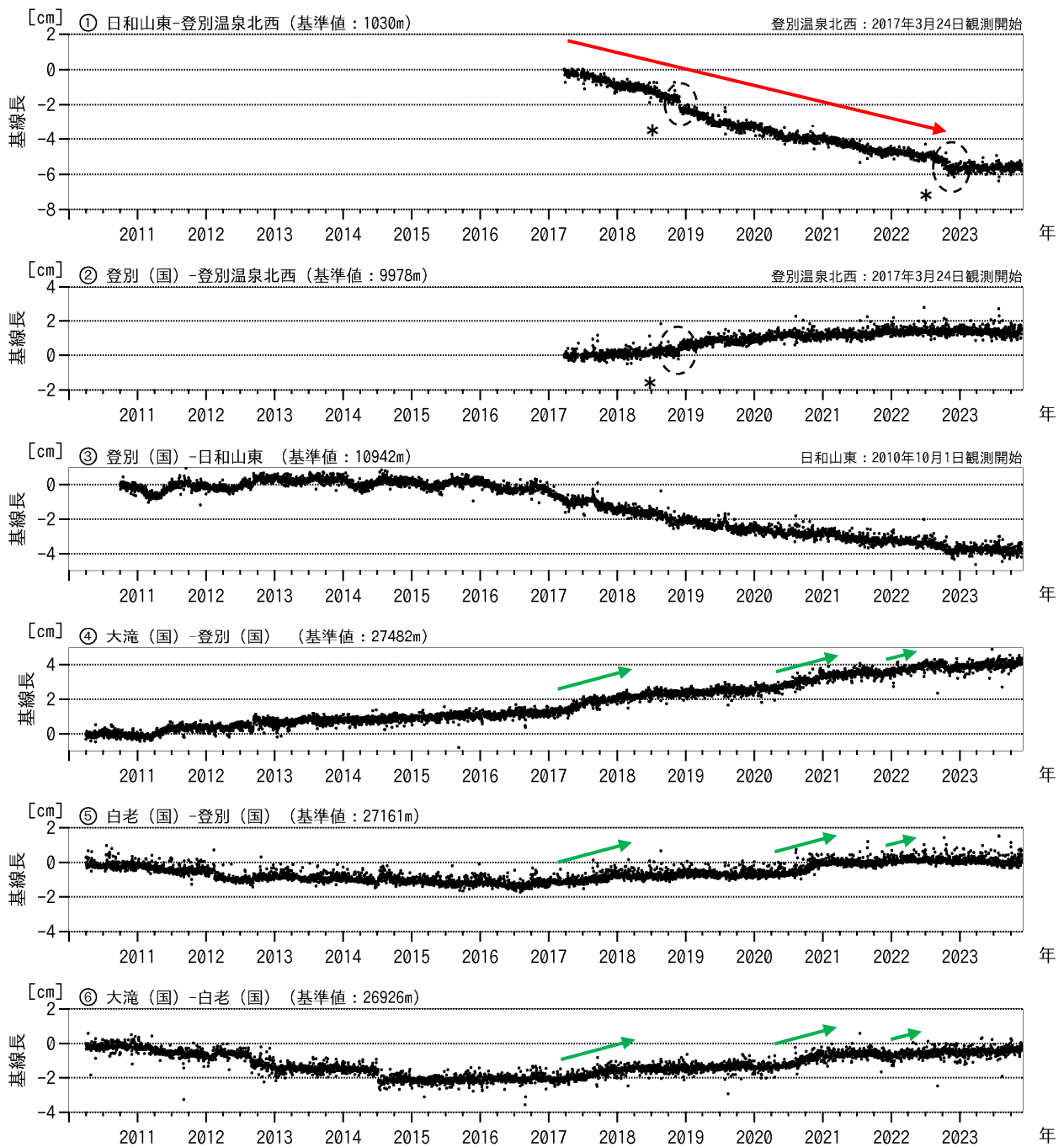
図9 倶多楽 GNSS連続観測による基線長変化（2010年4月～2023年11月）
