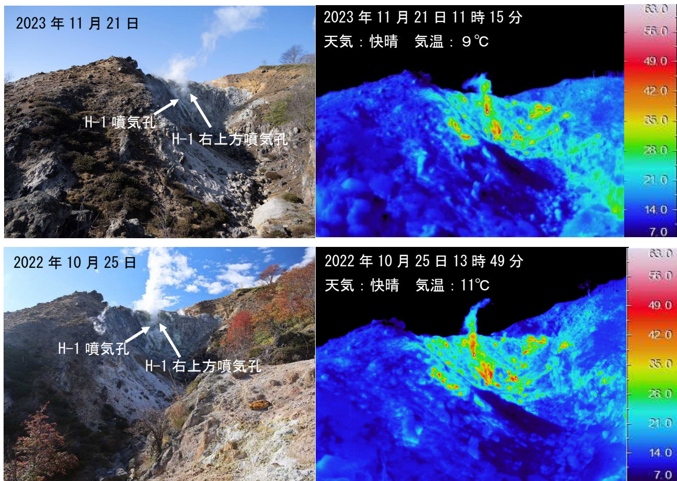
図4 倶多楽 日和山爆裂火口の地表面温度分布
