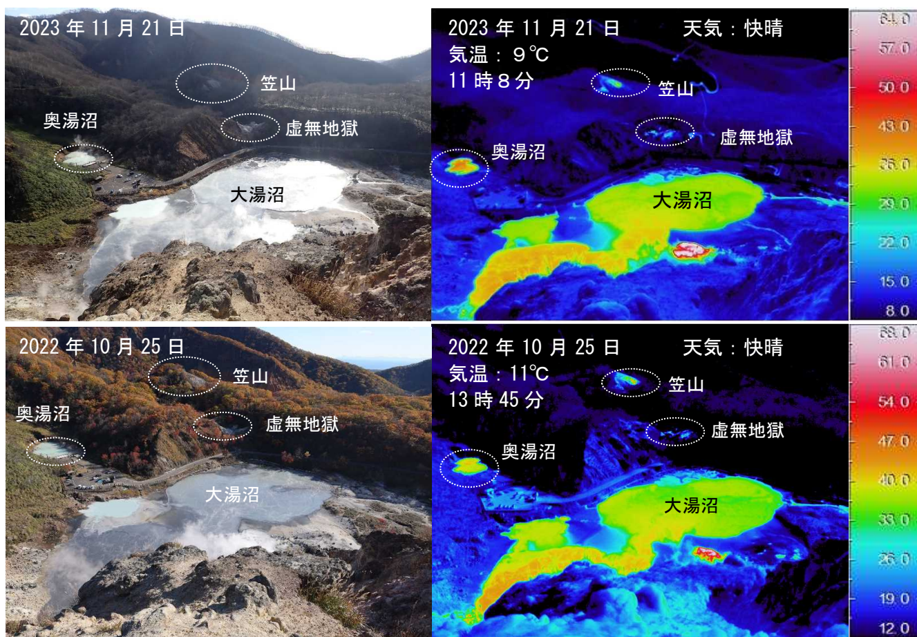
図6 倶多楽 笠山、虚無地獄、奥湯沼、大湯沼の地表面温度分布 北西側（図3の②：赤矢印）から撮影 ・前回の観測（2022年10月）と比べて、地表面温度分布に特段の変化は認められませんでした。
