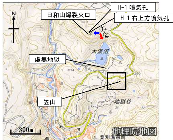
図3 倶多楽 周辺図と写真及び赤外熱映像の撮影方向（矢印） 図内の太枠線は図7の範囲を示します。
