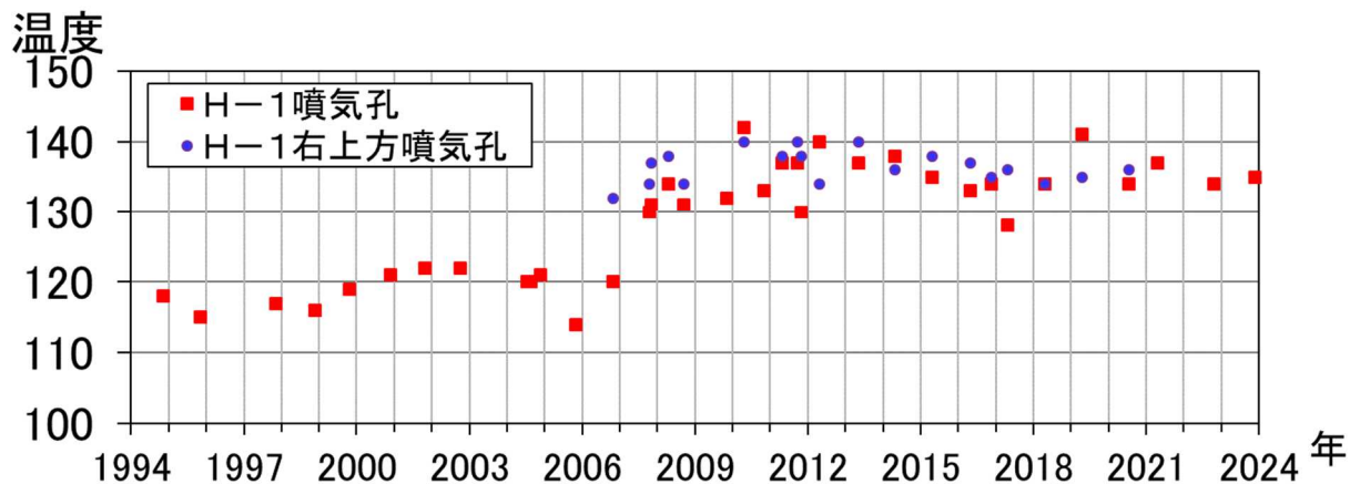
図5 倶多楽 日和山爆裂火口北西側噴気孔の噴気温度の推移（1994年～2023年） ・噴気温度は2007年以降、130℃以上の状態が継続しています。
