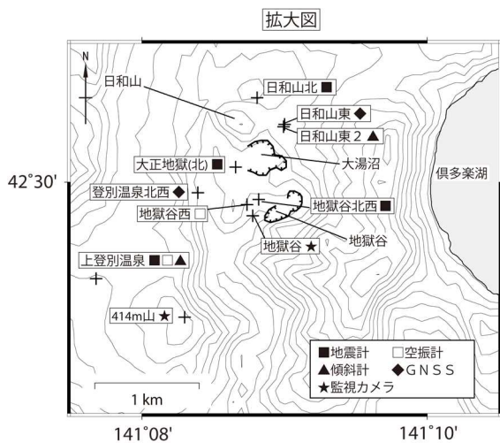
図10 倶多楽 観測点配置図
