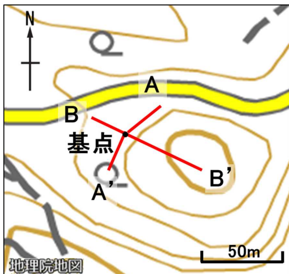
図7 倶多楽 笠山の地中温度観測の測線図 図内の赤線に沿って深さ50cmの地中温度を計測しています（図8）。
