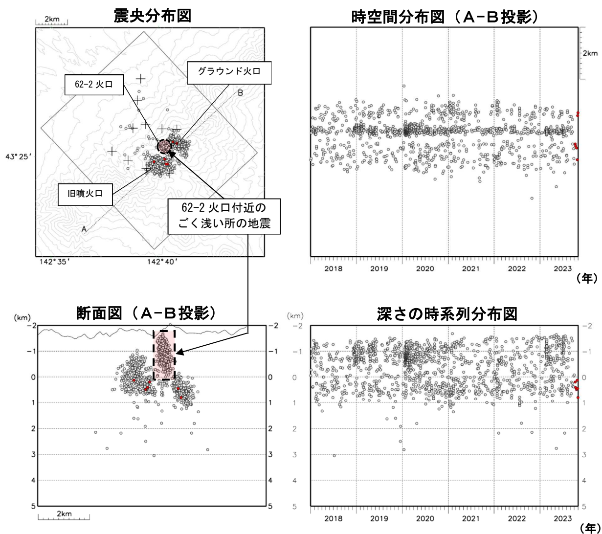
図4 十勝岳 火山性地震の震源分布（2018年1月～2023年10月）
