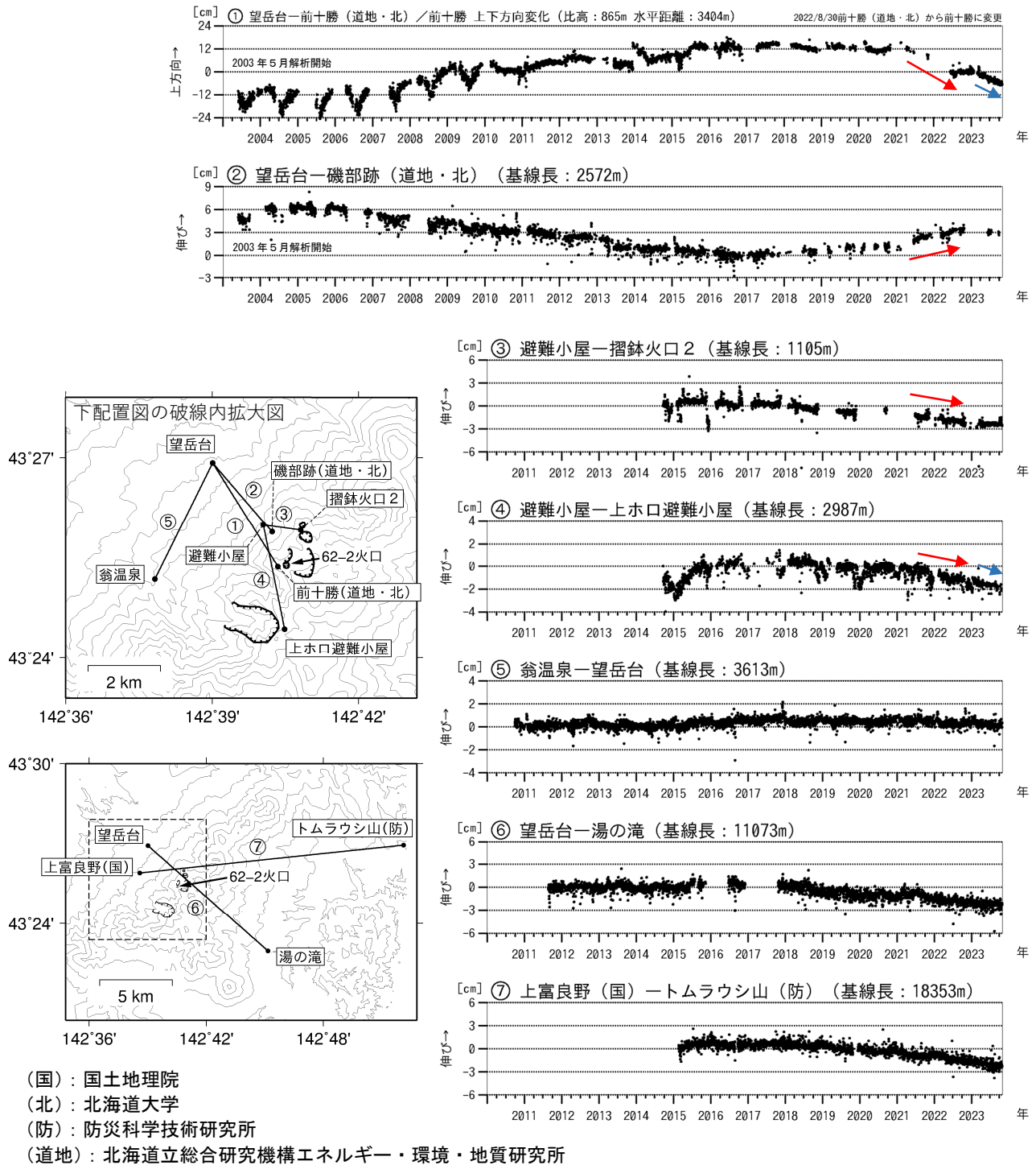
図5 十勝岳 GNSS連続観測による上下方向変化及び基線長変化（2003年5月～2023年10月）及び観測点配置図
