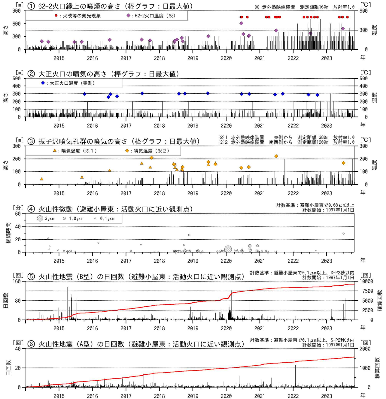
図2 十勝岳 火山活動経過図（2014年1月～2023年10月）
