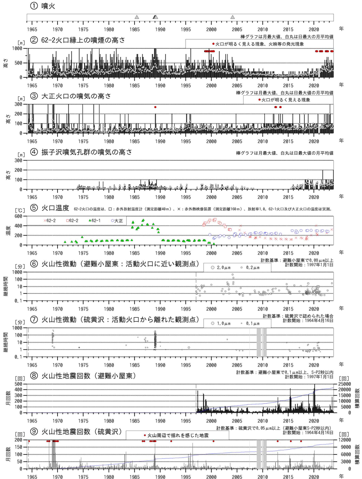
図1 十勝岳 火山活動経過図（1964年1月～2023年10月）
