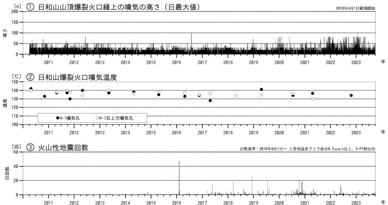
図2 倶多楽 火山活動経過図（2010年1月～2023年9月）
