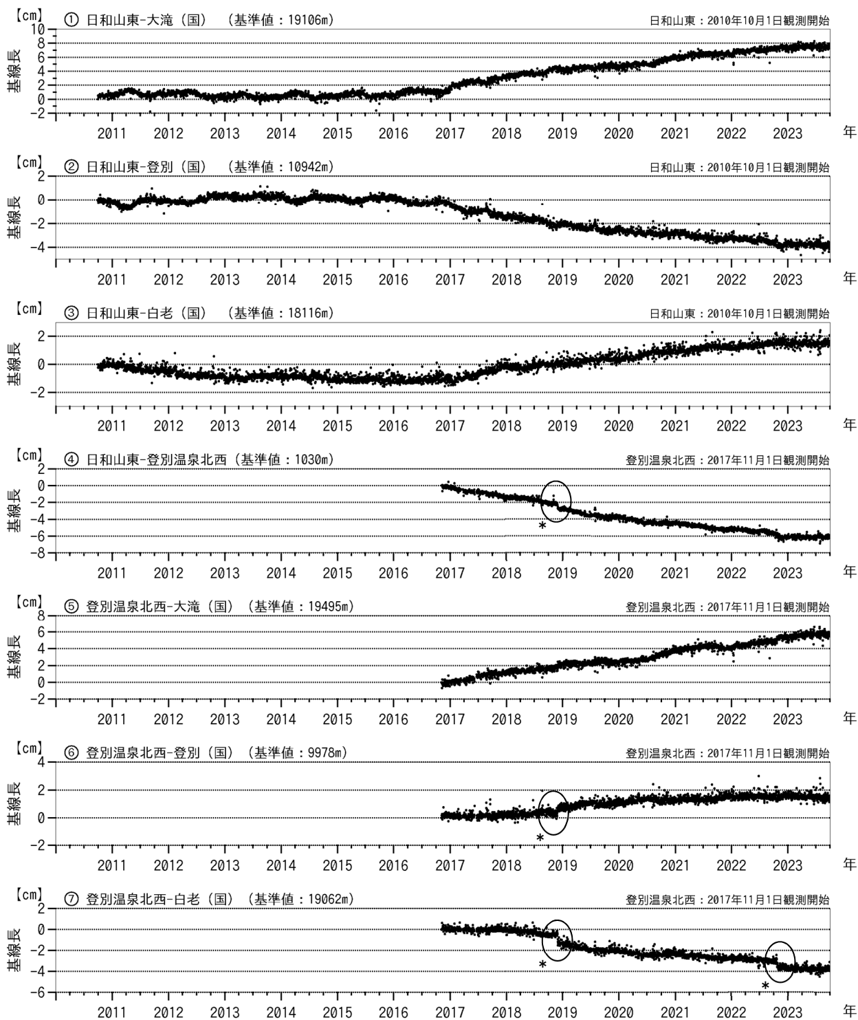
図3 倶多楽 GNSS連続観測による基線長変化 (2010年10月～2023年9月)
