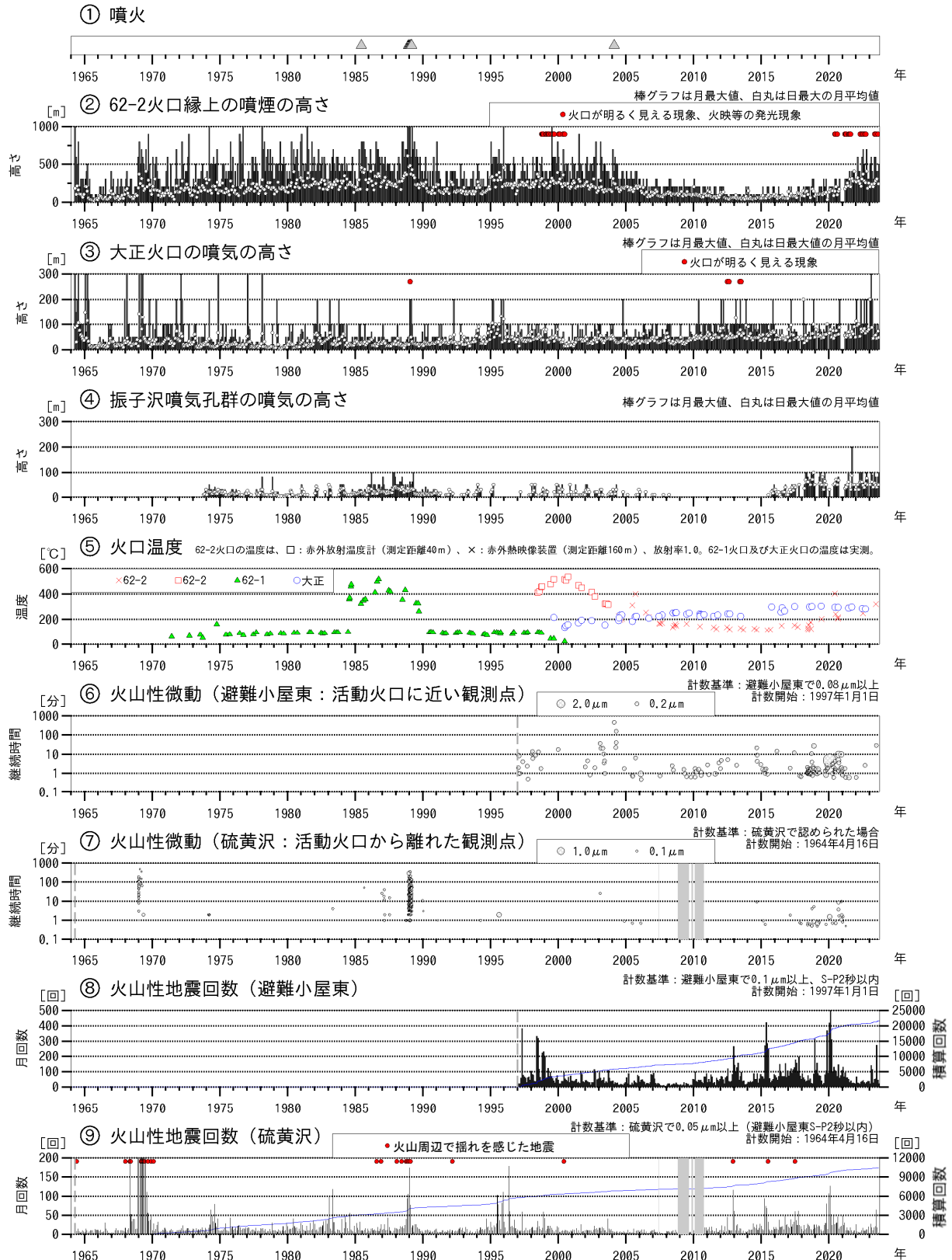
図1 十勝岳 火山活動経過図（1964年1月～2023年9月）
