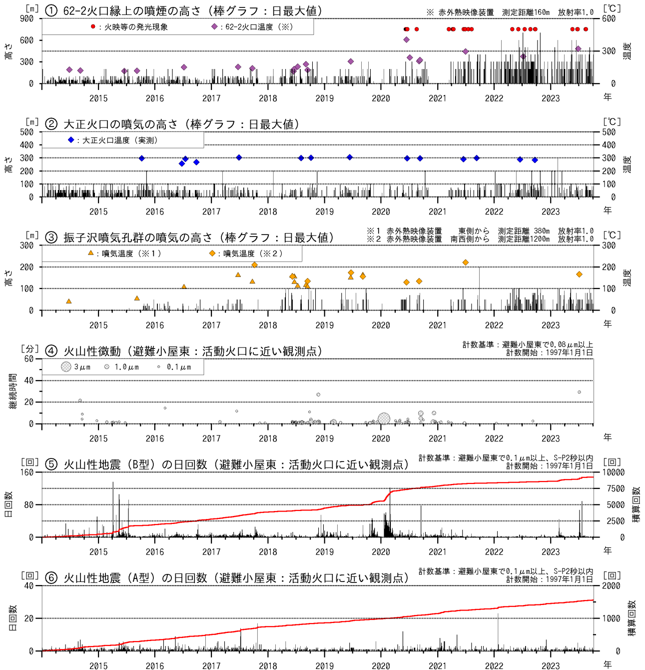
図2 十勝岳 火山活動経過図（2014年1月～2023年9月）
