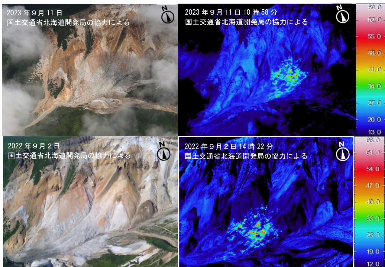
図6 十勝岳 赤外熱映像装置による旧噴火口の地表面温度分布
