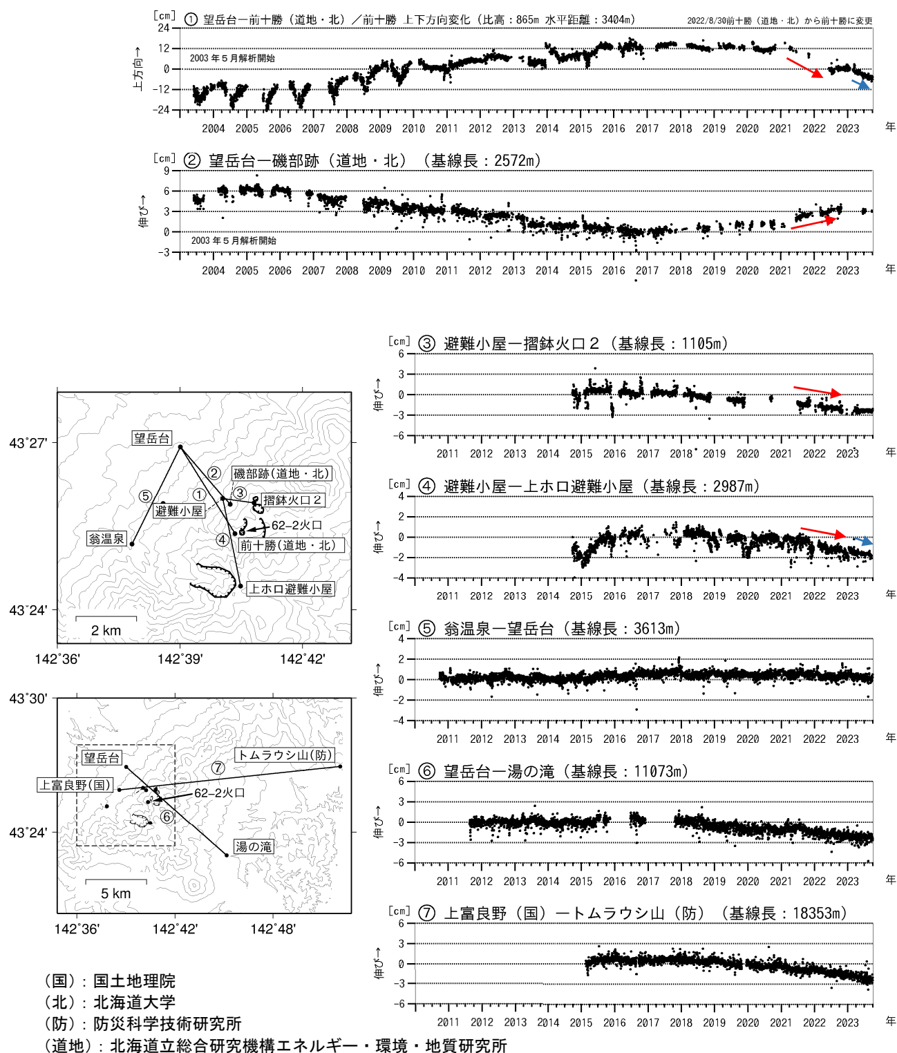
図8 十勝岳 GNSS連続観測による上下方向変化及び基線長変化（2003年5月～2023年9月）及び観測点配置図
