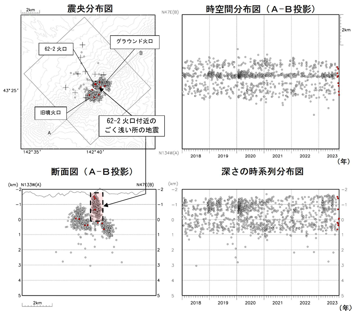
図7 十勝岳 火山性地震の震源分布（2018年1月～2023年9月）
