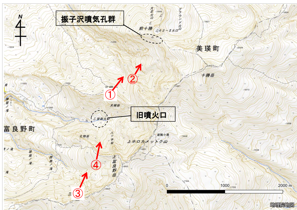
図4 十勝岳 火口周辺図と写真及び熱映像の撮影位置（番号）及び撮影方向（矢印）
